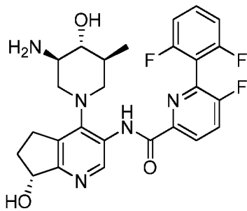
Соединение 1
