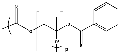
Формула Ye
