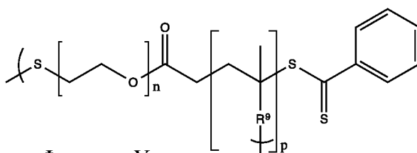
Формула Yc
