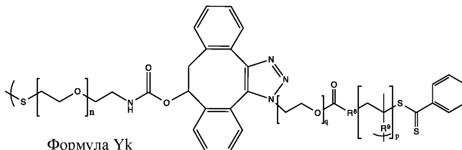
Формула Yj
