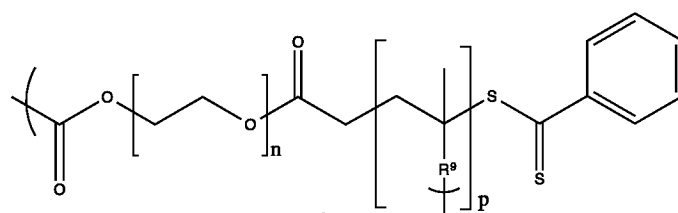
Формула Yf
