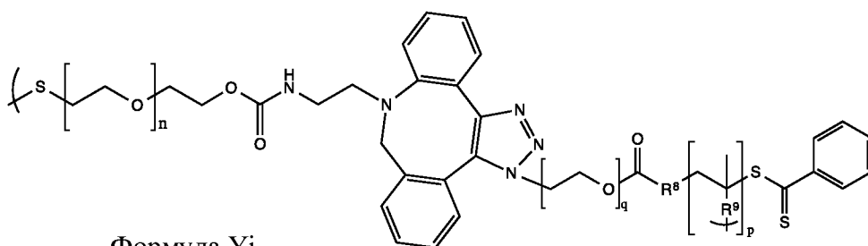
Формула Yi
