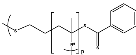
Формула Yd
