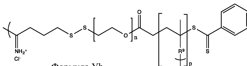
Формула Yb
