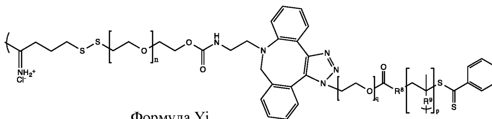
Формула Yj
