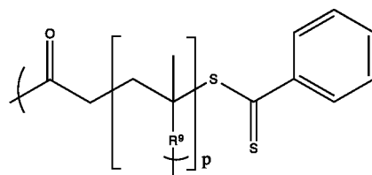
Формула Yg
