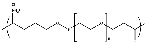
Формула Ya
