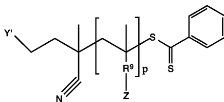
Формула Y'-CMP
