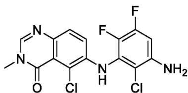
6-((3-Амино-2-хлор-5,6-дифторфенил)амино)-5-хлор-3-метилхиназолин-4(3H)-
