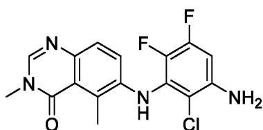
6-((3-Амино-2-хлор-5,6-дифторфенил)амино)-3,5-диметилхиназолин-4(3H)-он
