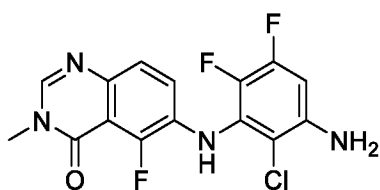
6-((3-Амино-2-хлор-5,6-дифторфенил)амино)-5-фтор-3-метилхиназолин-4(3H)-он
