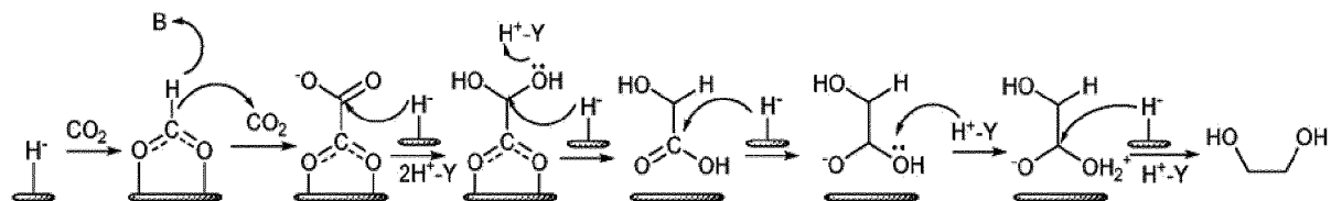
ФИГ. 3D) Оксалатный путь
