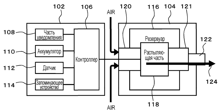
100A Фиг. 1А
