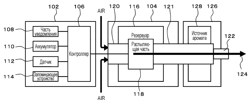
100B Фиг. 1В
