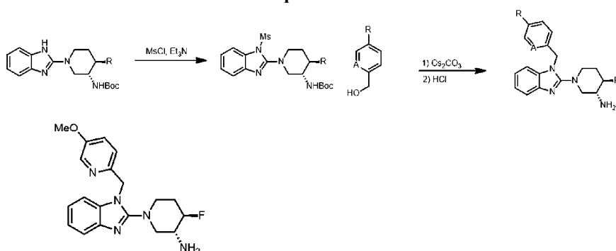
Схема 13 Химия переноса мезилата
