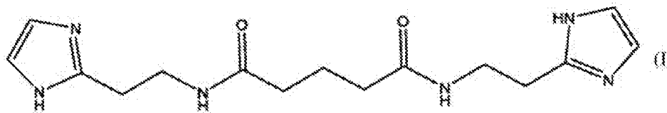
N,N'-бис-[2-(1H-имидазол-4-ил)этил]пентандиамид
