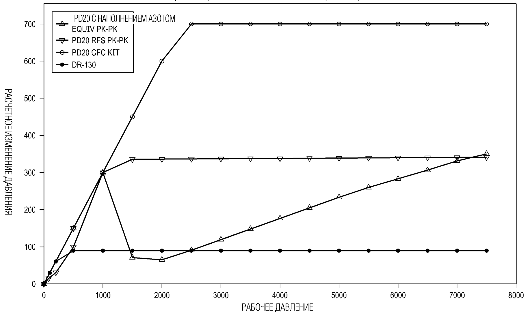
Сравнительные данные для сред/размеров, при диаметре поршня 5,5 (140 мм) × длине хода 12 дюймов (305 мм)
