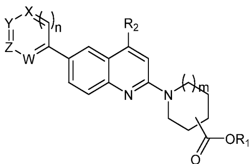
Формула I
