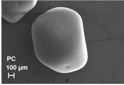
Увеличение = 50 X Сигнал A = SE2 Рабочий отрезок = 19,0 мм Высокое напряжение = 5,00Кв Вакуумная камера = 2,62e-006 мбар
