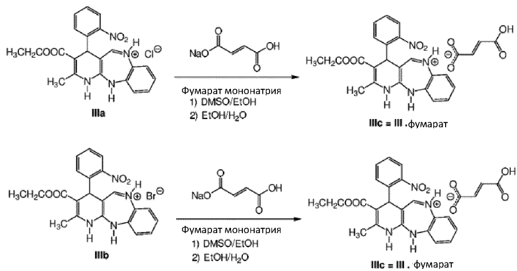
Фиг. 6. Получение фумаратной соли из JM-20 (IIIc).
