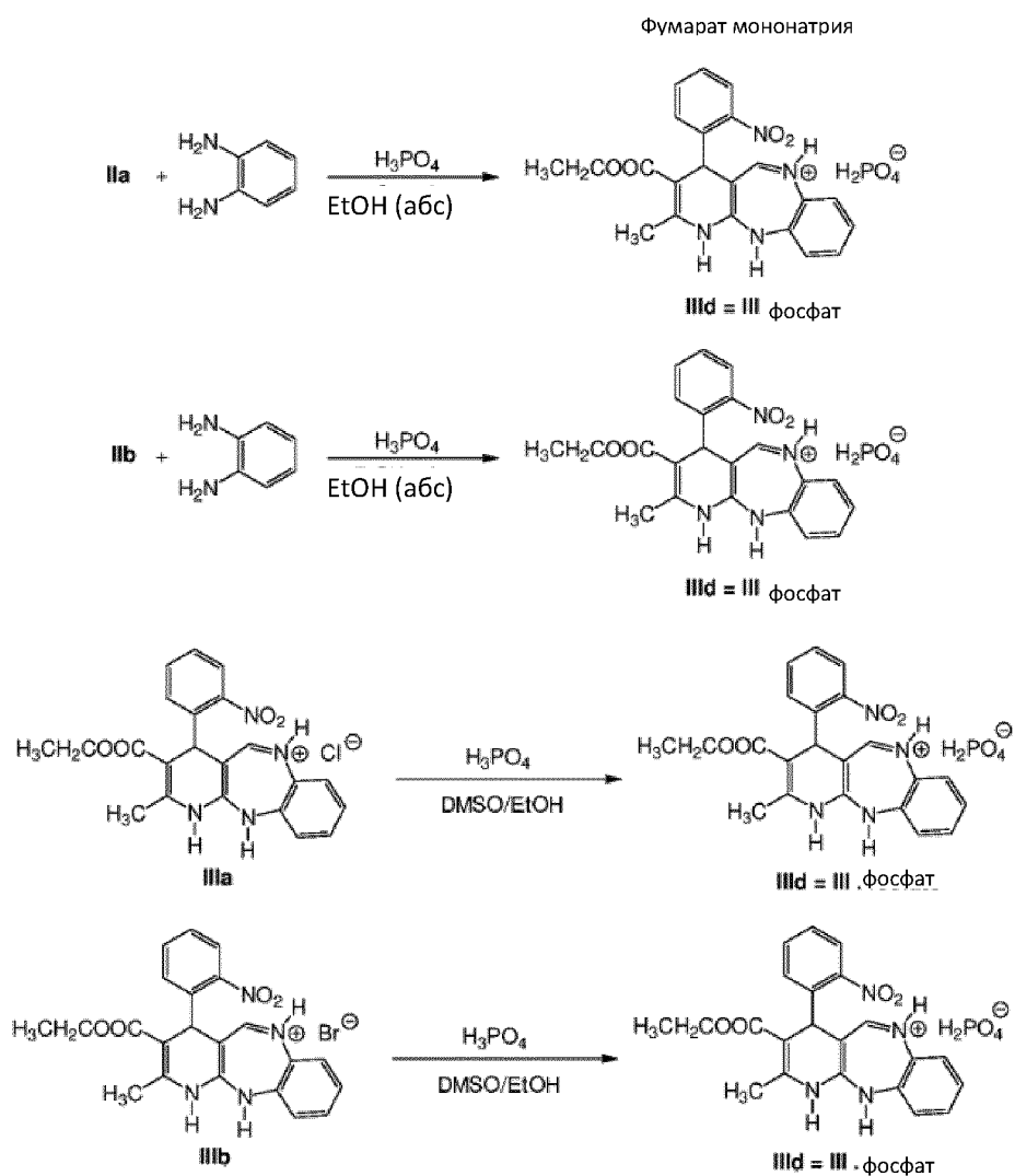
Фиг. 7. Получение фосфатной соли из JM-20 (III d).
