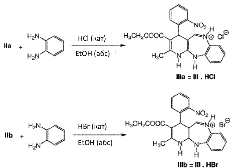
Фиг. 5. Схема получения соединения III и его галогенидов
