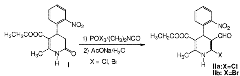
Фиг. 1. Схема получения IIa и IIb
