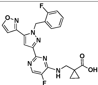
I-358
