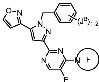
Формула IVa
