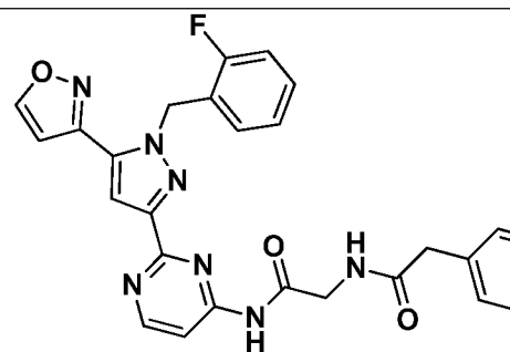
I-597
