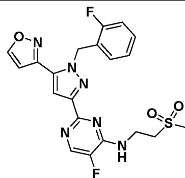
I-487
