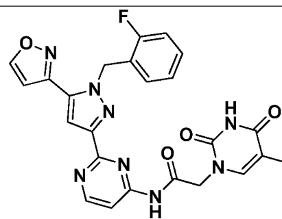
I-571
