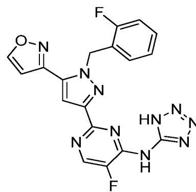
I-276
