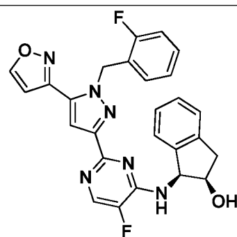
I-395
