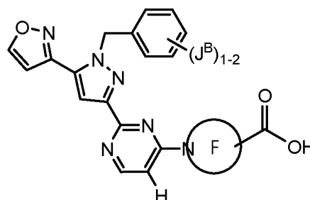
Формула Vb,
