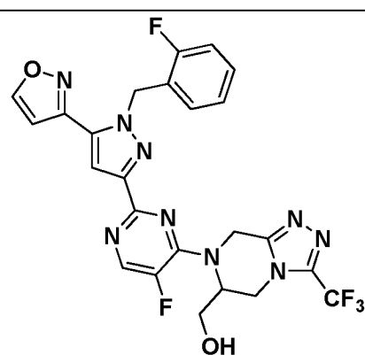
I-633
