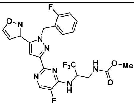
I-568
