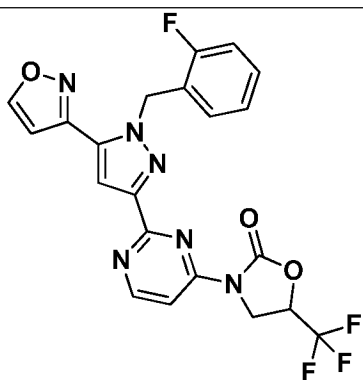
I-482
