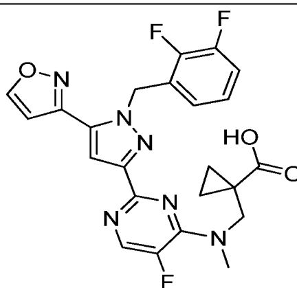
I-304
