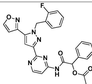
I-565
