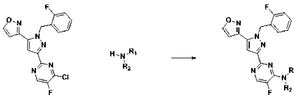
Промежуточное соединение 1
