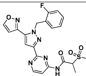
I-587
