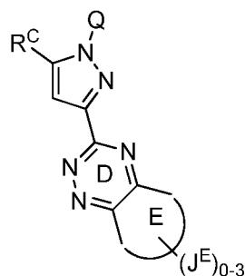
Формула VI'a;
