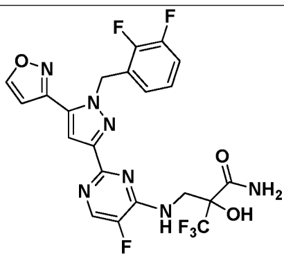
I-522
