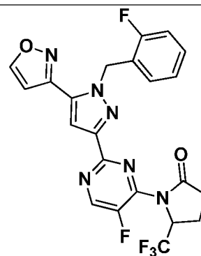
I-501
