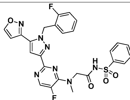
I-361
