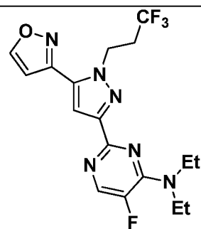
I-517
