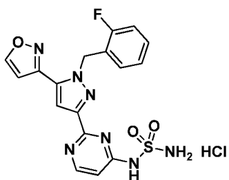
I-456
