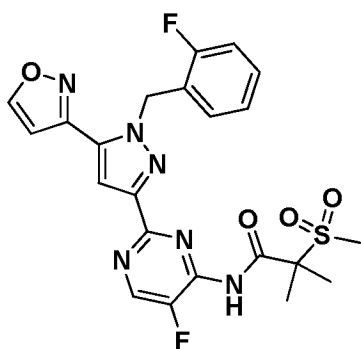
I-582
