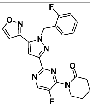
I-506
