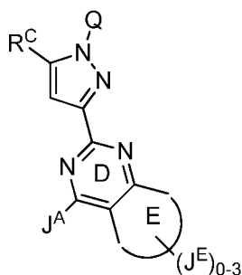
Формула V'a
