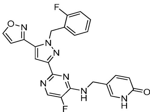
I-278
