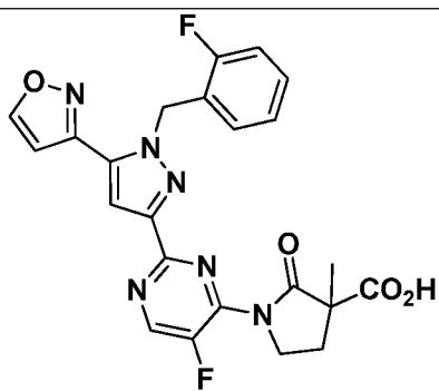
I-604
