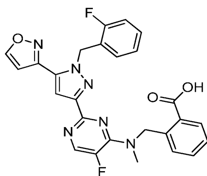
I-279
