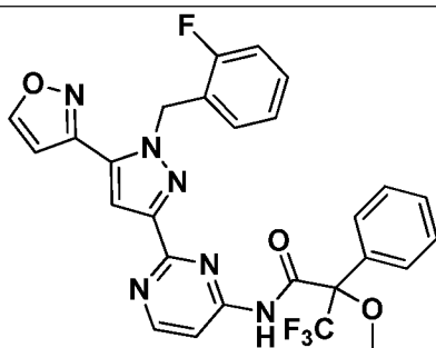
I-572
