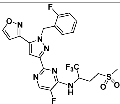
I-588
