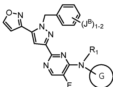
Формула VIa
