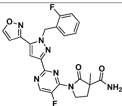
I-606
