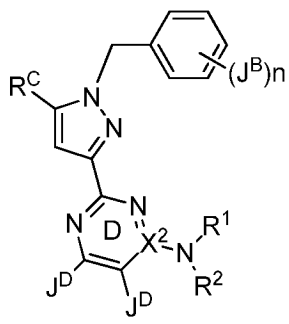
Формула IV'б
