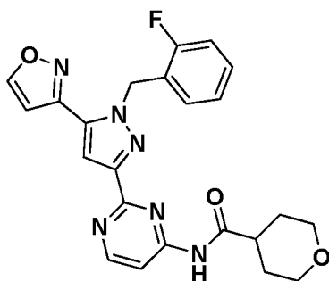
I-574
