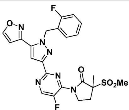
I-526
