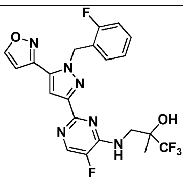
I-634
