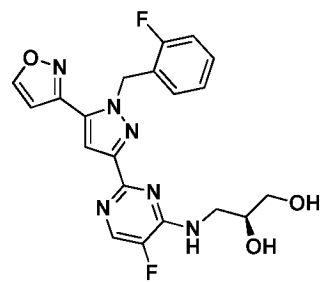
I-313
