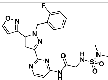
I-586
