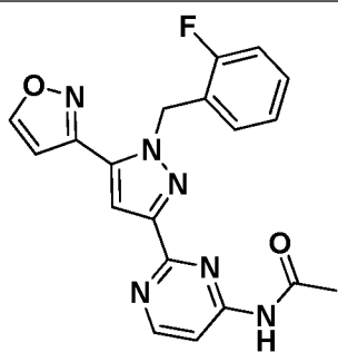
I-524
