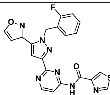
I-549
