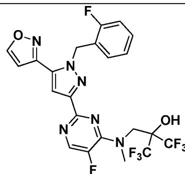
I-529
