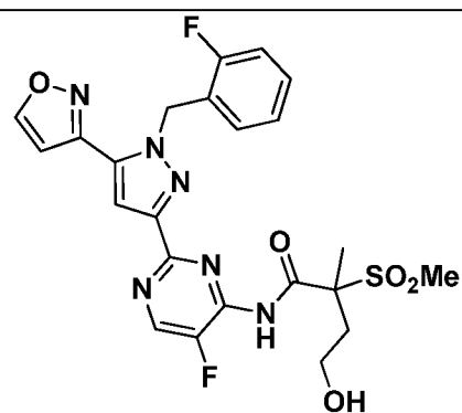
I-527
