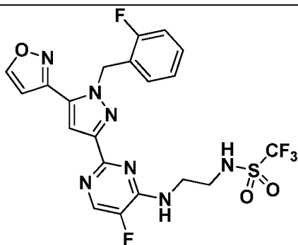
I-392
