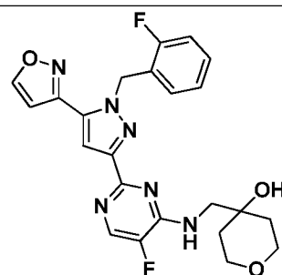
I-397
