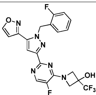
I-396
