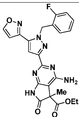
I-420
