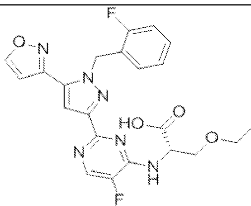
I-302
