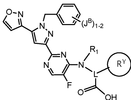
Формула IXa
