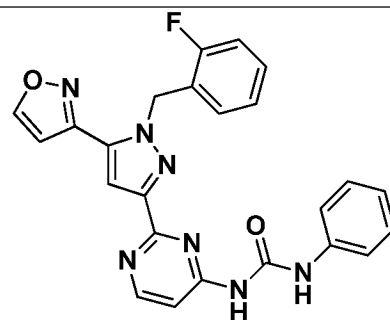
I-583
