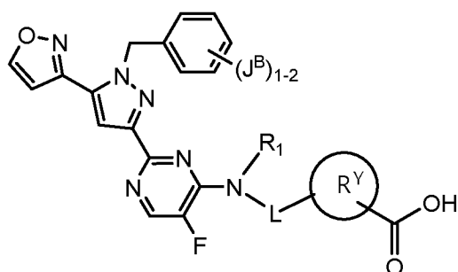
Формула Xa
