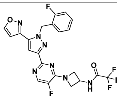
I-387
