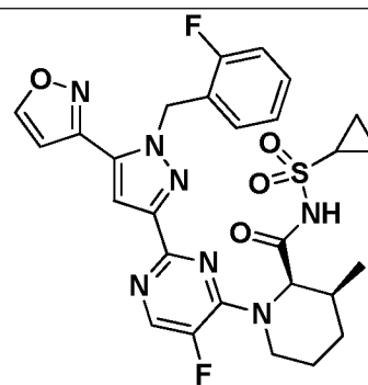
I-331
