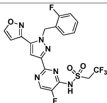
I-609
