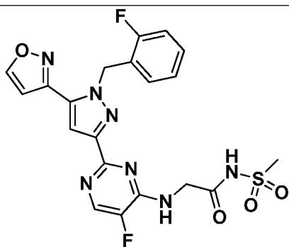
I-546
