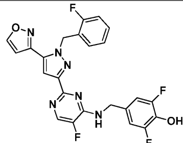
I-317
