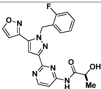
I-576
