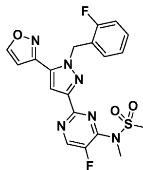
I-629
