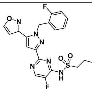
I-611
