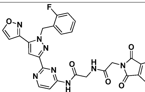
I-602
