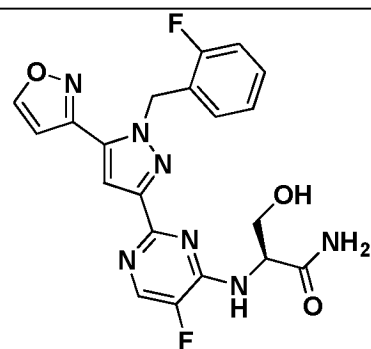
I-335
