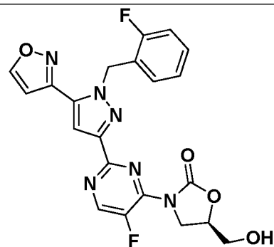
I-575
