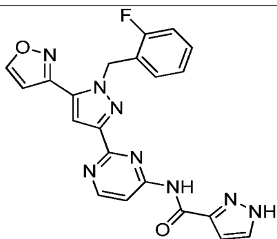
I-386
