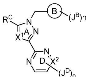
Формула II'b
