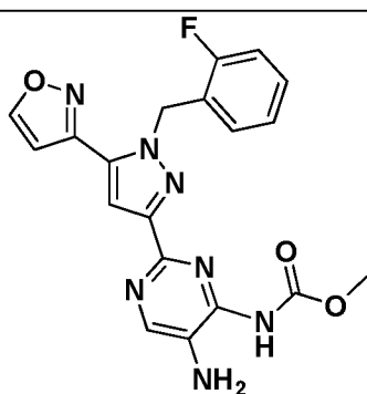
I-542
