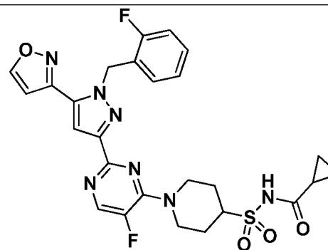
I-423
