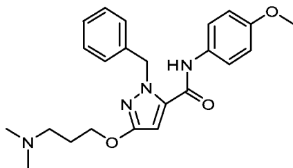
CFM-1571 (см. публикацию патента WO2000027394)
