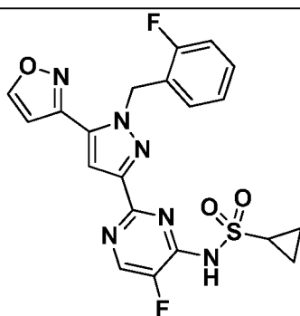
I-610
