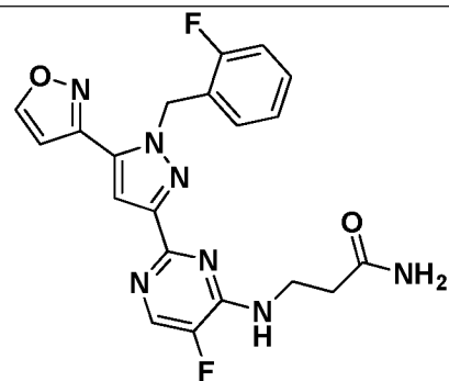
I-581
