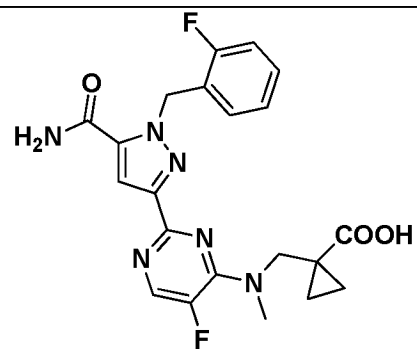
I-481
