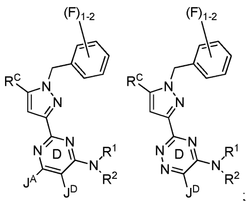
X'b, XI'b
