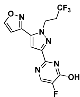
I-507
