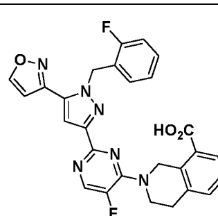
I-337
