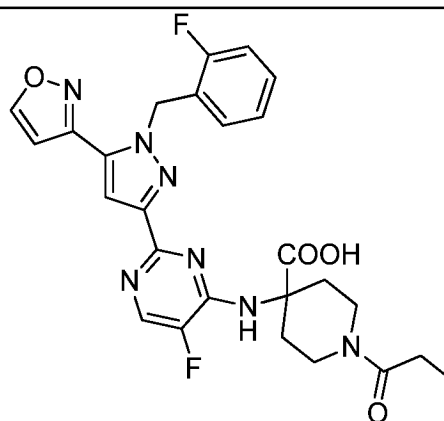
I-128
