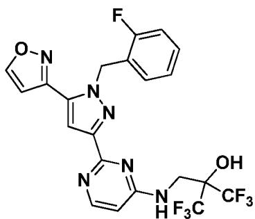
I-500
