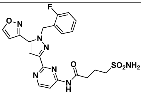
I-484
