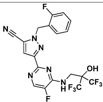
I-474
