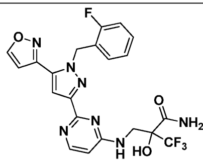
I-627
