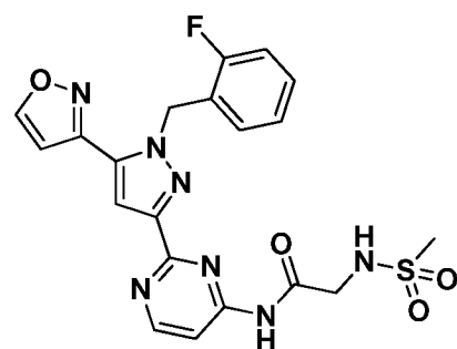
I-543
