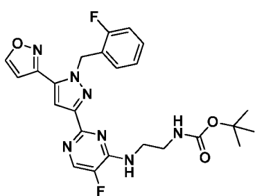
I-390
