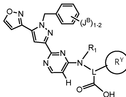
Формула IXb
