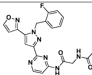
I-535
