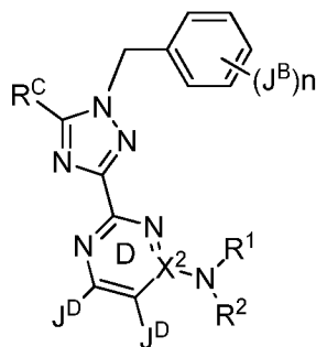
Формула IV'с.
