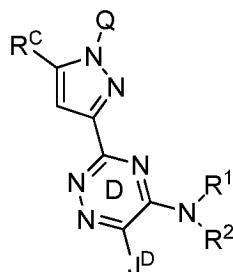
Формула X'a.
