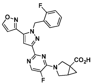
I-312
