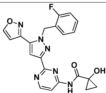
I-478
