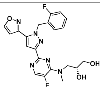
I-319
