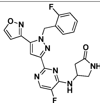
I-485
