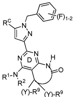
Формула XIX'b
