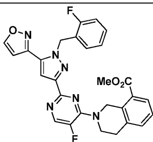
I-338
