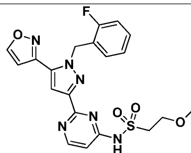
I-479
