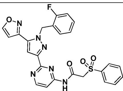
I-592
