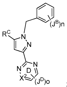
Формула III'б
