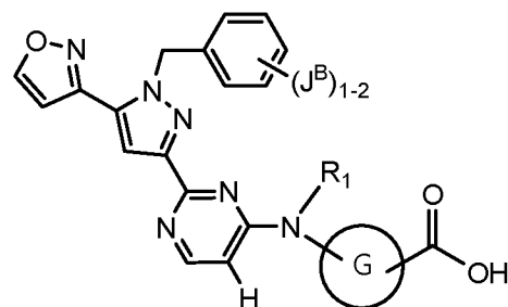
Формула VIIb
