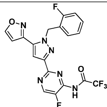
I-463
