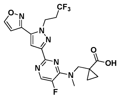
I-523
