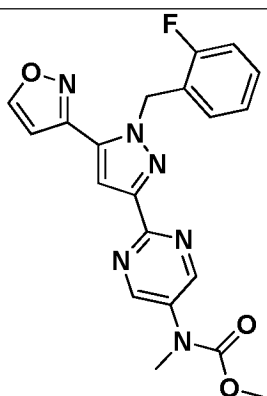
I-630
