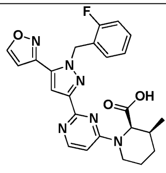
I-333
