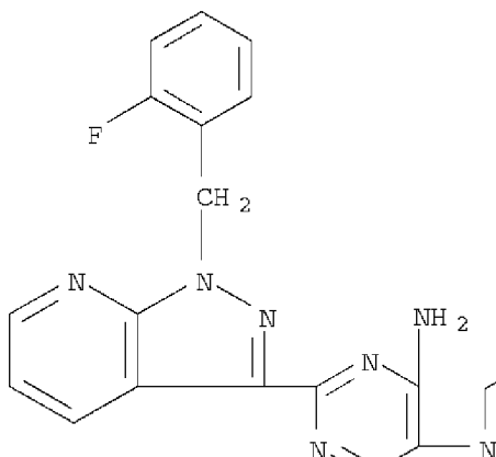
Этрицигуат (описан в WO 2003086407)
