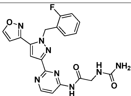
I-584
