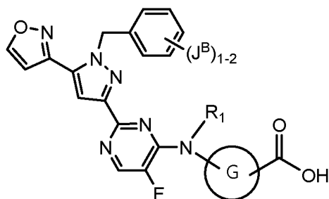
Формула VIIa
