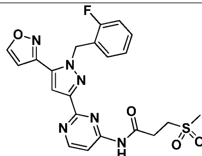
I-573
