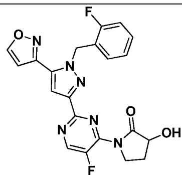
I-615
