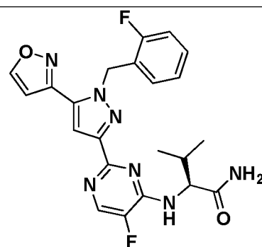
I-537
