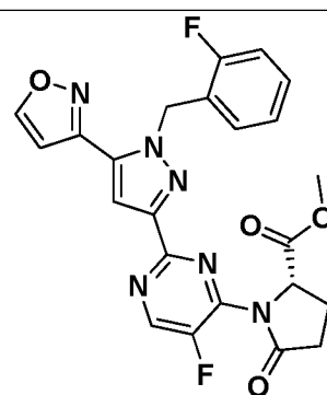
I-401
