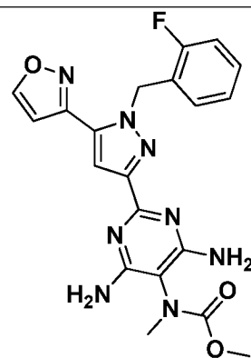
I-621
