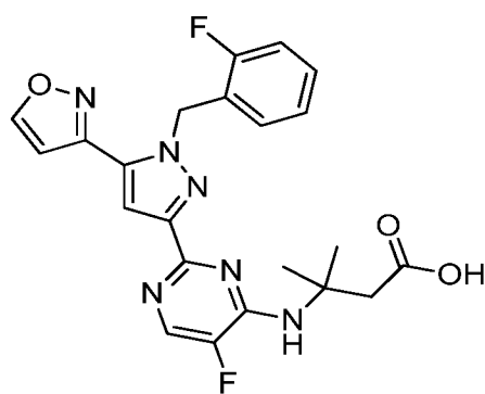
I-277
