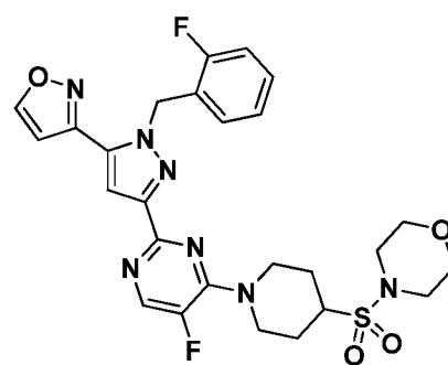
I-423
