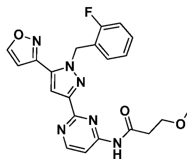
I-547
