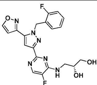
I-316
