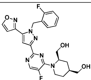
I-318
