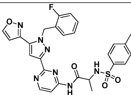
I-548
