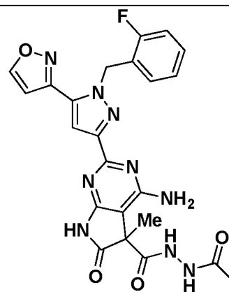
I-623
