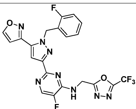
I-608
