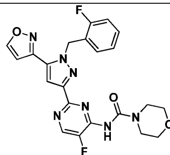
I-477
