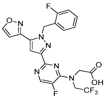
I-273
