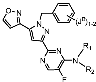
Формула XIa
