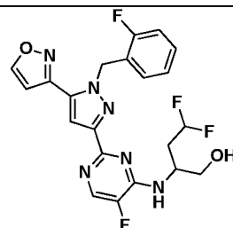
I-399
