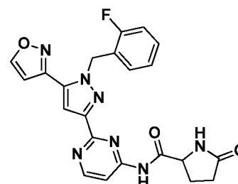
I-459
