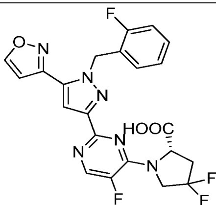
I-301
