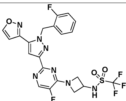
I-388
