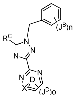
Формула III'с.
