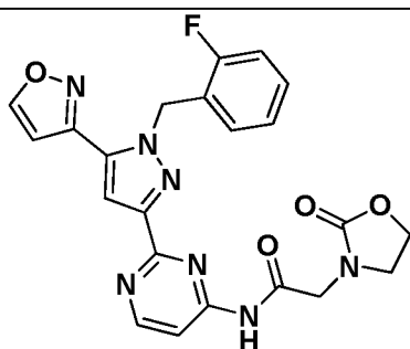
I-600
