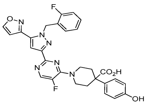
I-297
