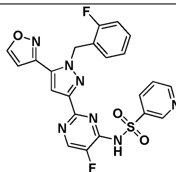
I-625
