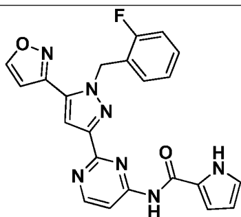
I-550
