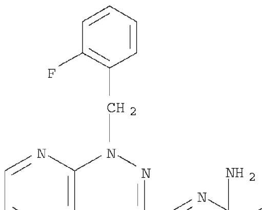
CFM-1571 (см. публикацию патента WO2000027394)
