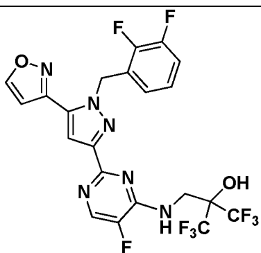
I-488
