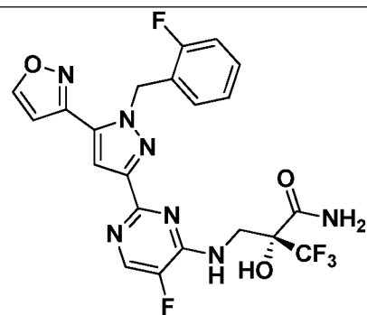
I-531
