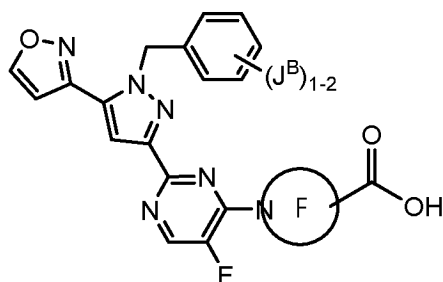
Формула Va
