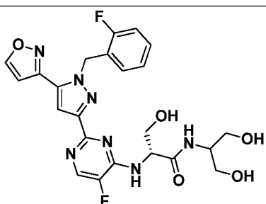
I-336
