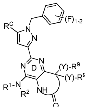
Формула XIX'd.
