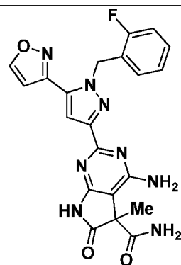
I-421
