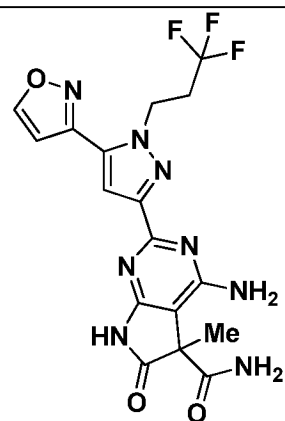
I-619
