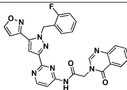
I-601
