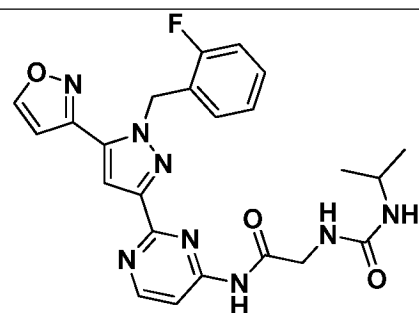
I-585
