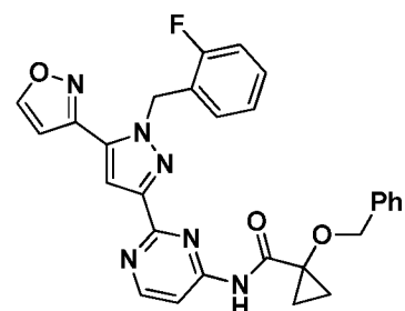
I-461
