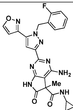
I-422
