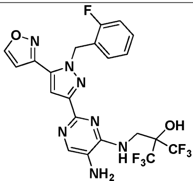
I-484
