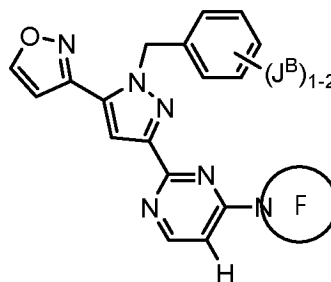
Формула IVb,
