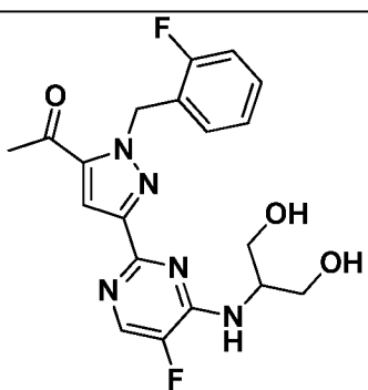
I-462
