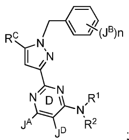
Формула V'b
