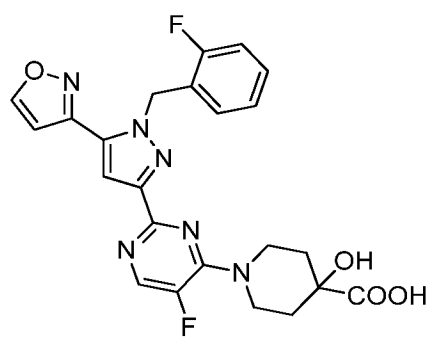
I-300
