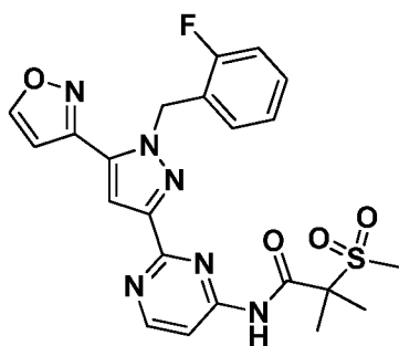
I-580
