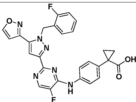
I-360
