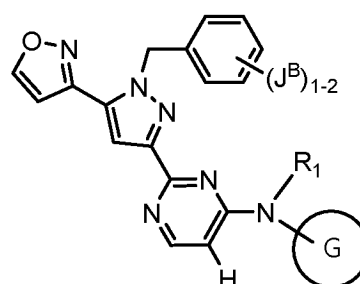
Формула VIb,
