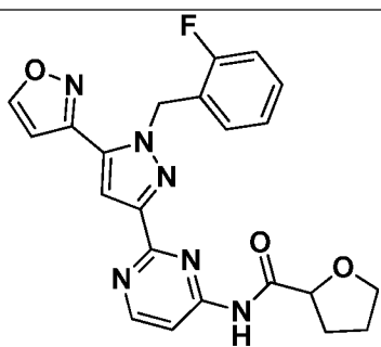
I-570
