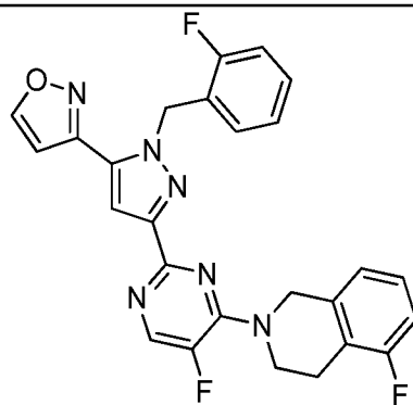
I-128
