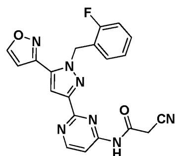
I-579
