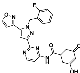
I-458
