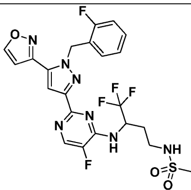
I-544
