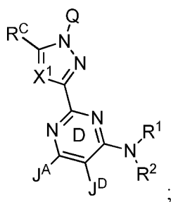
Формула IV'a
