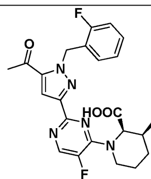
I-463
