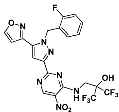
I-483
