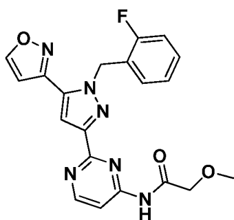
I-528
