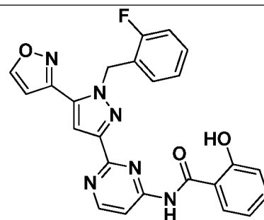
I-577
