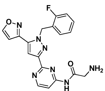
I-520
