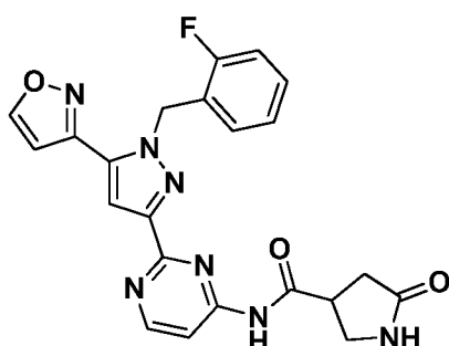
I-462
