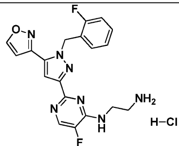
I-391
