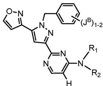
Формула XIb;
