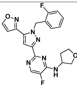
I-578
