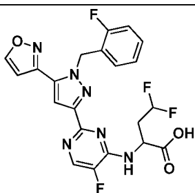
I-398
