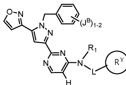
Формула VIIb
