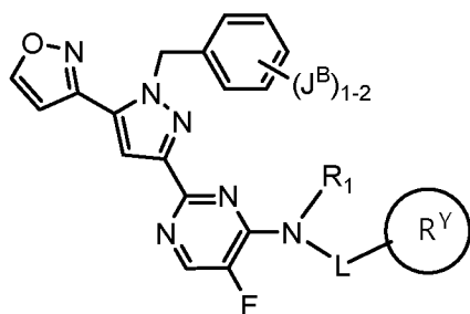
Формула VIIa
