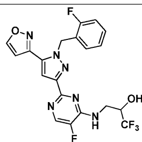
I-337
