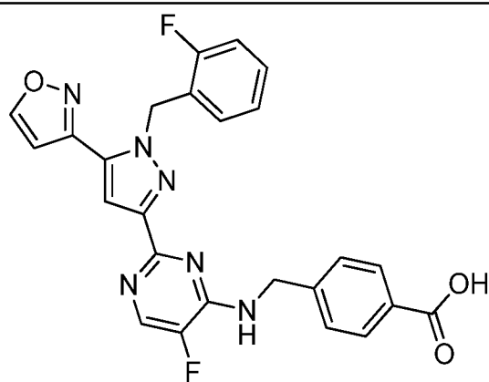
I-280
