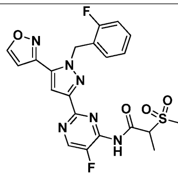
I-589
