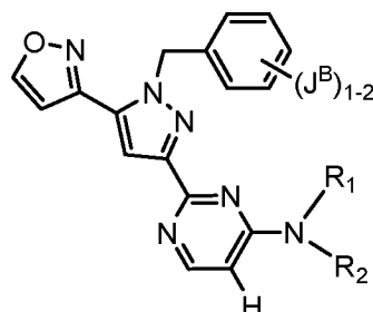
Формула XIb
