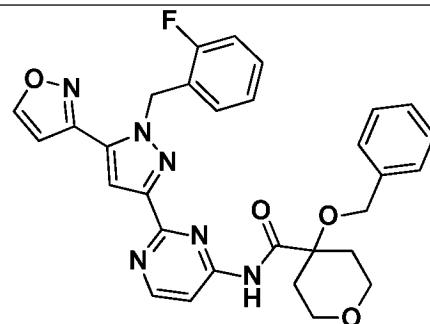
I-525
