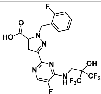
I-476
