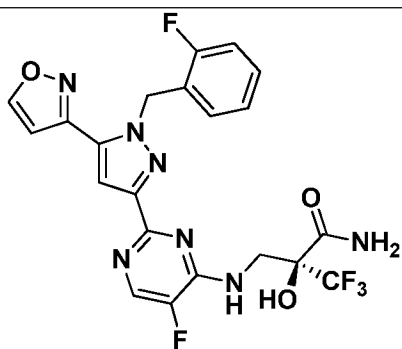
I-530
