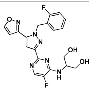
I-315
