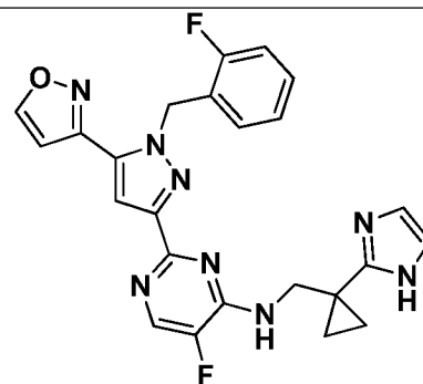
I-567
