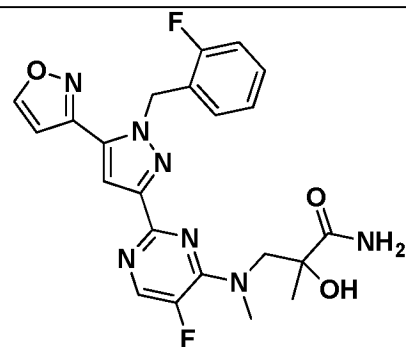
I-393
