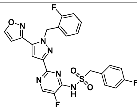
I-607
