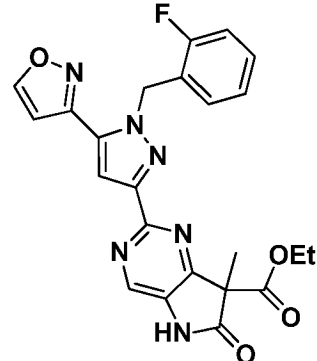
I-617
