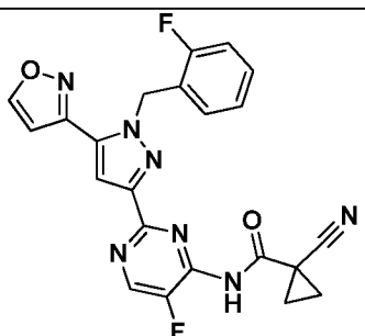
I-460
