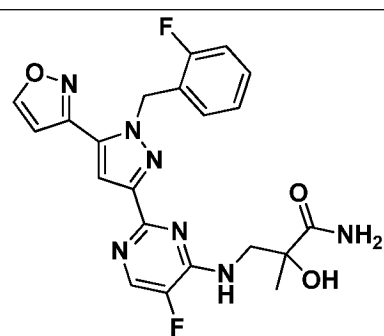
I-389
