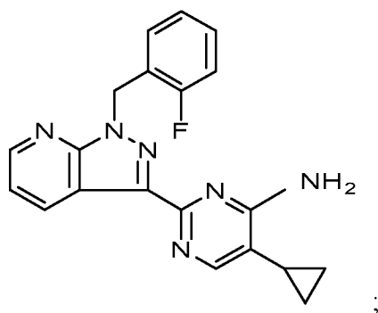
BAY 41-8543 (описан в DE19834044)
