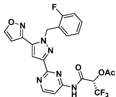
I-475
