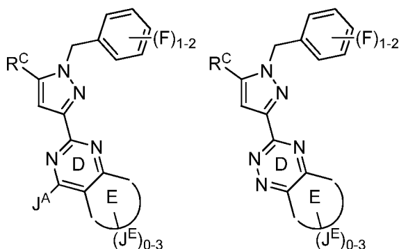
Формула VI'b Формула VII'b
