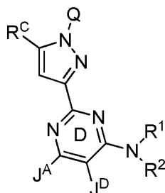
Формула XIX'a
