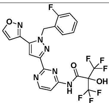
I-400
