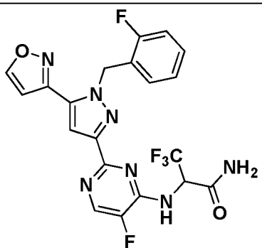
I-540
