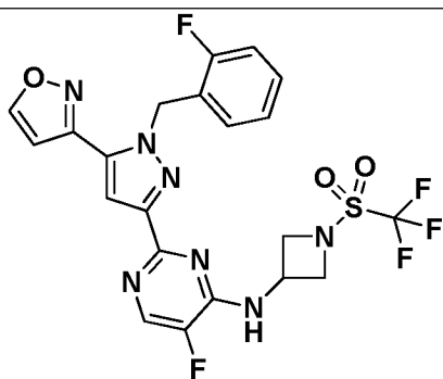
I-394
