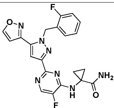
I-538
