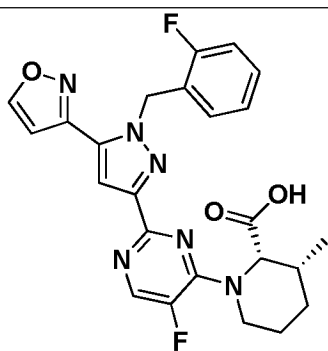
I-330
