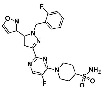
I-364
