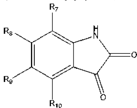
(формула IV),
