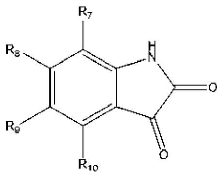
(формула IV),
