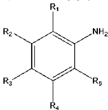
(формула I),
