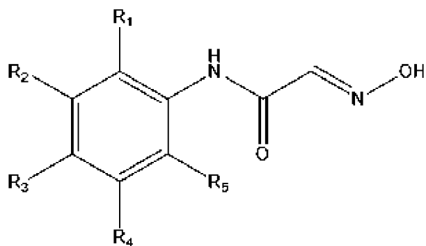
(формула II),
