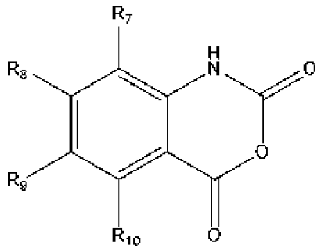
(формула V),
