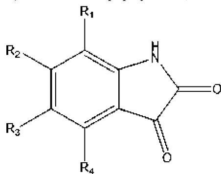
(формула III),
