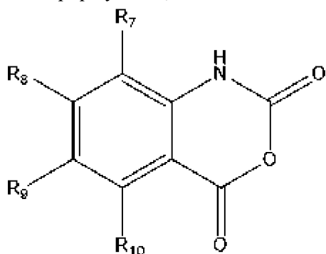
(формула V),
