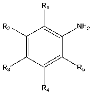
(формула I),
