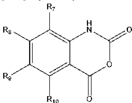
(формула V),
