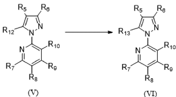
Схема 16.
