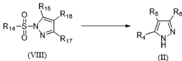
Схема 11.
