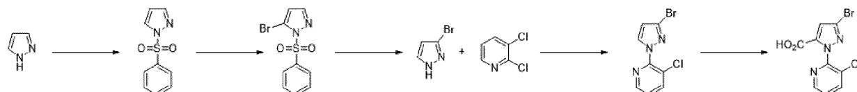
Схема 4.
