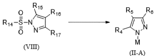
Схема 12.
