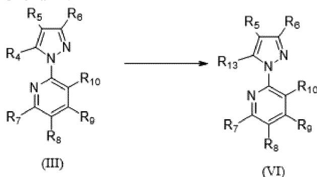
Схема 14.
