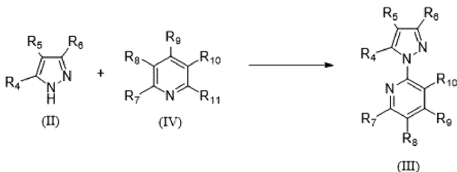
Схема 13.
