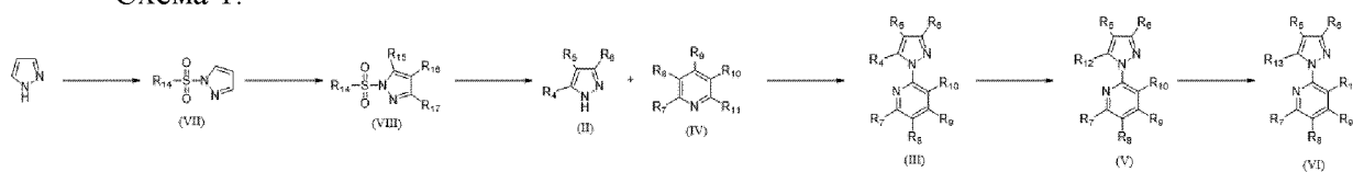
Схема 1.
