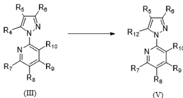
Схема 15.
