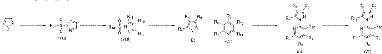
Схема 2.
