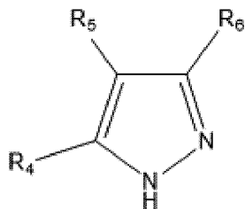
(формула II),
