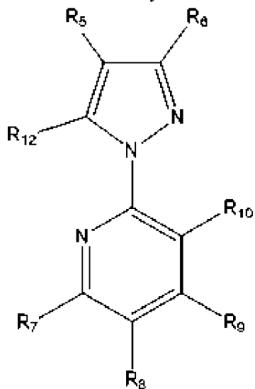
(формула V),
