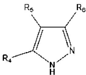
(формула II),
