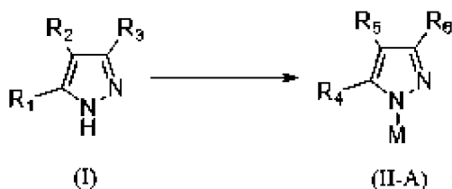
Схема 6.
