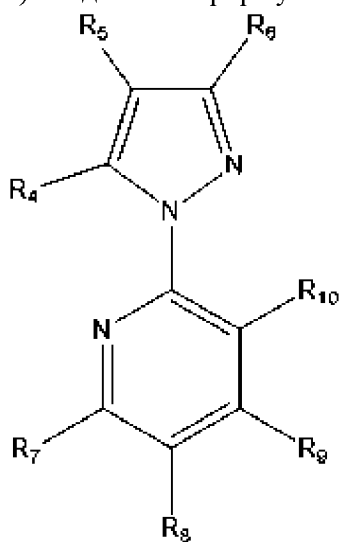
(формула III),
