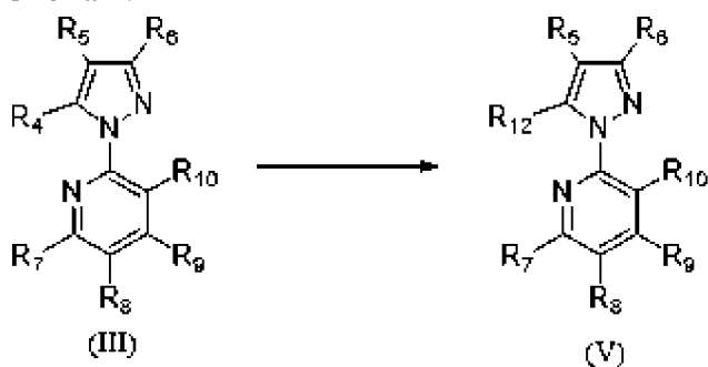
Схема 9.
