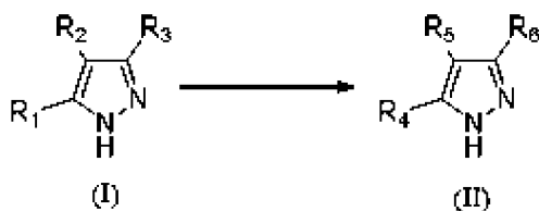
Схема 5.
