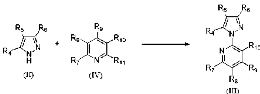
Схема 7.
