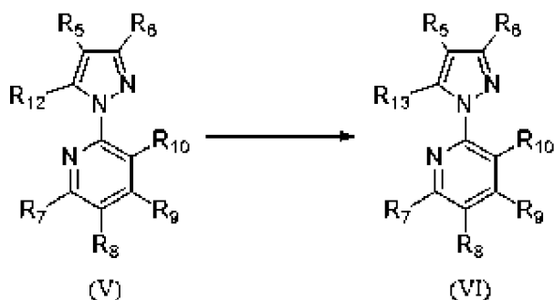
Схема 10.
