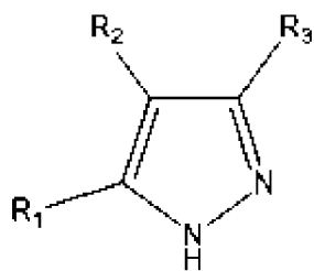
(формула I),
