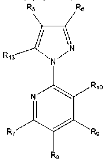
(формула VI),
