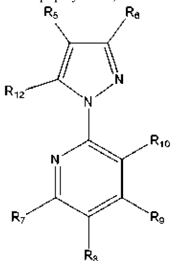
(формула V),
