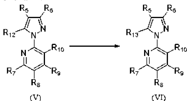
Схема 11.
