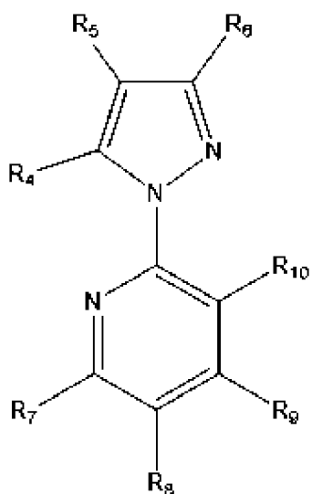
(формула III),
