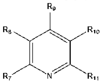
(формула IV),
