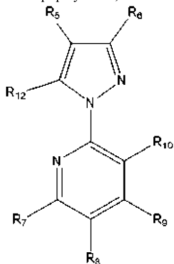
(формула V),
