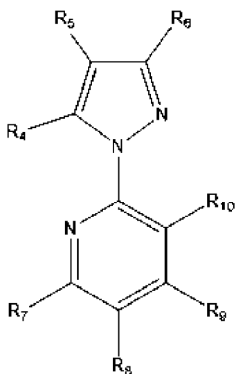
(формула III),
