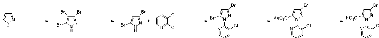
Схема 2.
