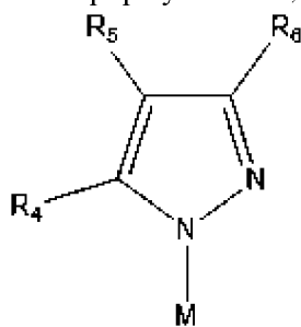
(формула II-A),
