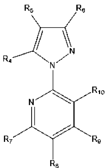
(формула III),
