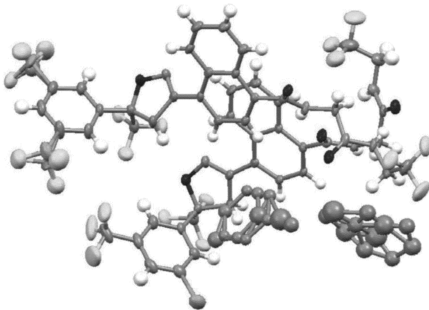
Фиг. 9: Структура монокристалла (S)-афоксоланера
