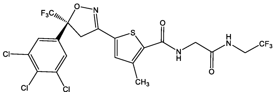
Лотиланер
