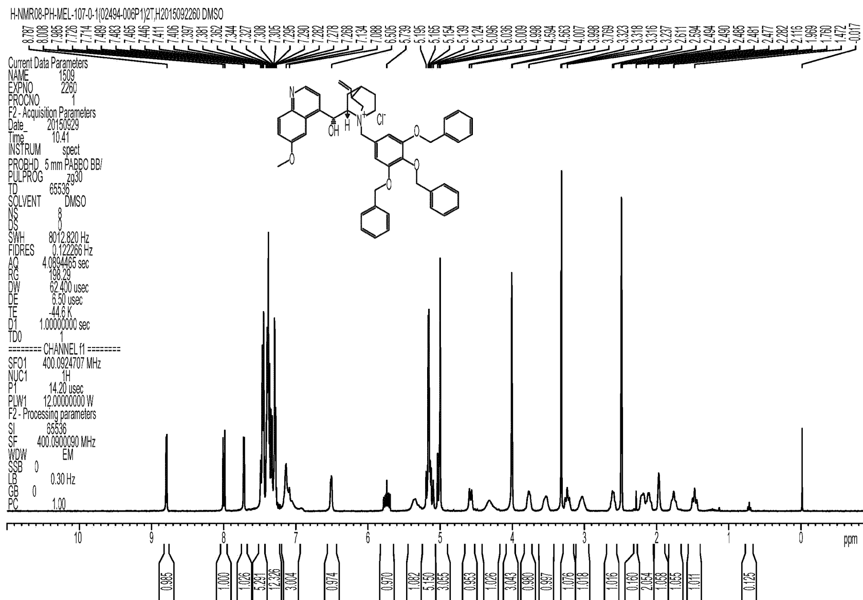
Фиг. 1: ^1\text{H} ЯМР спектр хирального катализатора межфазного переноса (IIIa-13-1), полученного в Примере 1, в \text{DMSO-d}_6
