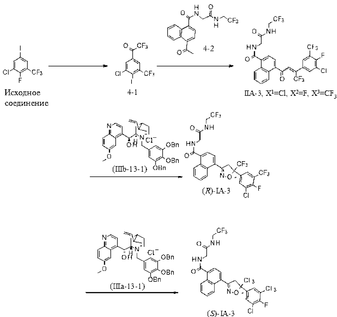
Схема 4
