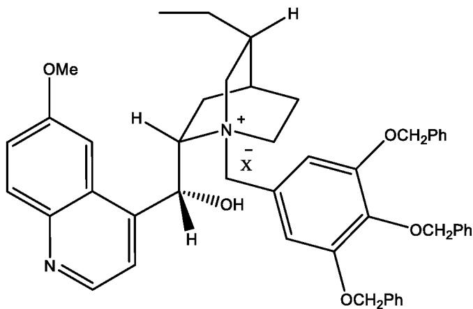
(Ша-13-2)
