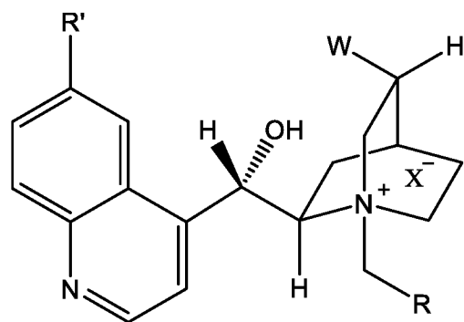
(IIIb)
