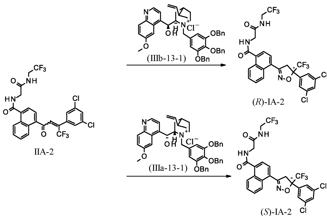
Схема 3
