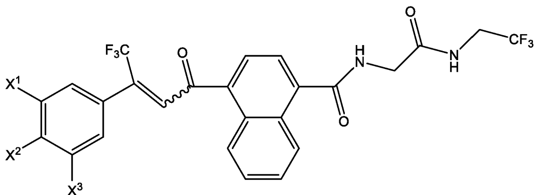
(IIA)
