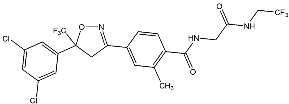
Флураланер
