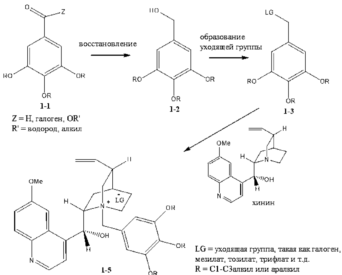
Схема 1
