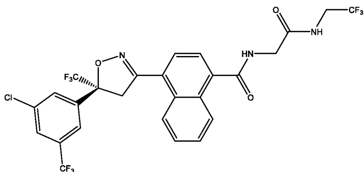
(S)-афоксоланер
