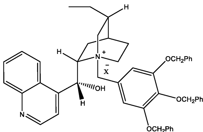
(Ша-13-4)
