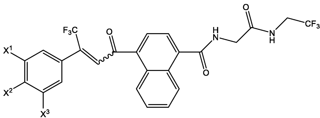
(IIA)
