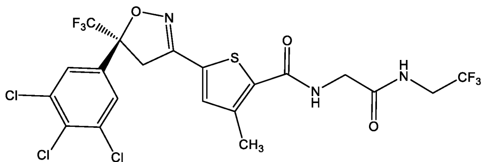
Лотиланер
