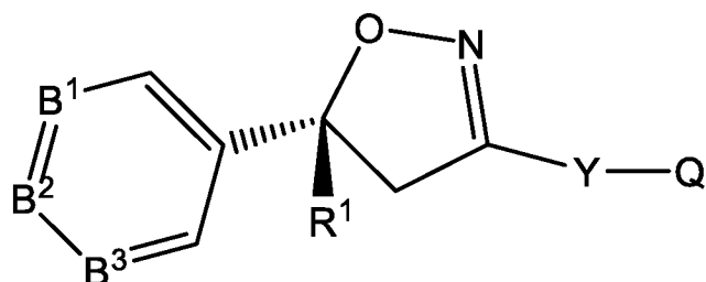
(R)-I
