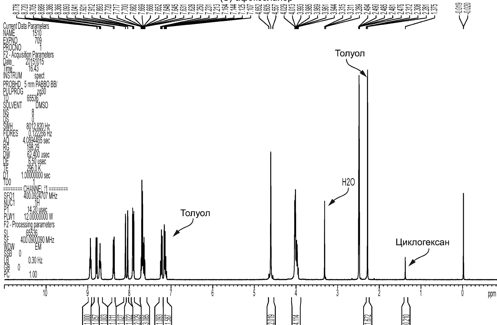
Фиг. 3: 1 H ЯМР спектр (S)-афоксоланера, полученного в Примере 7, в ДМСО-d 6
