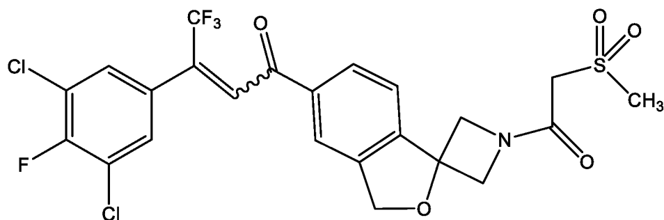
(ПС-1)
