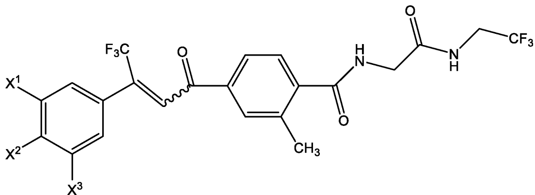
(IIБ)
