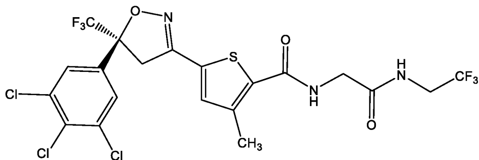
Лотиланер
