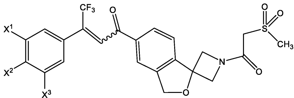
(IIС)
