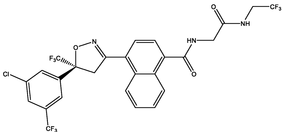
( S )-афоксоланер
