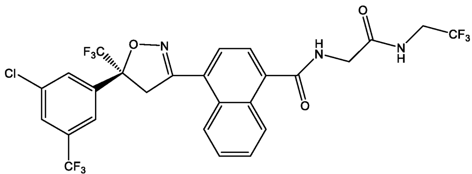
( S )-афоксоланер
