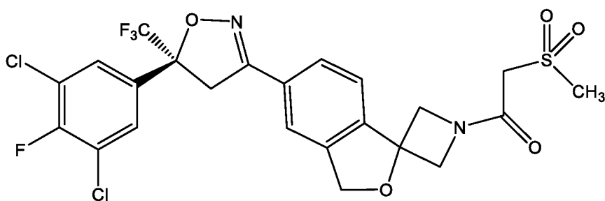
Сароланер
