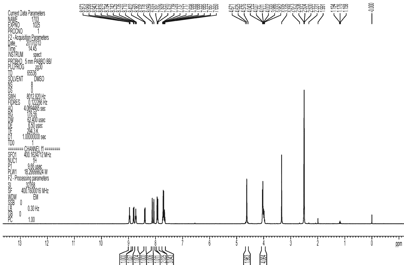
Фиг. 4: 1 H ЯМР спектр афоксоланера (рацемического) в ДМСО-d 6
