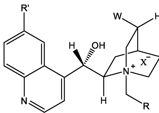
(IIIb)
