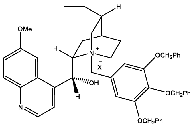
(Ша-13-2)
