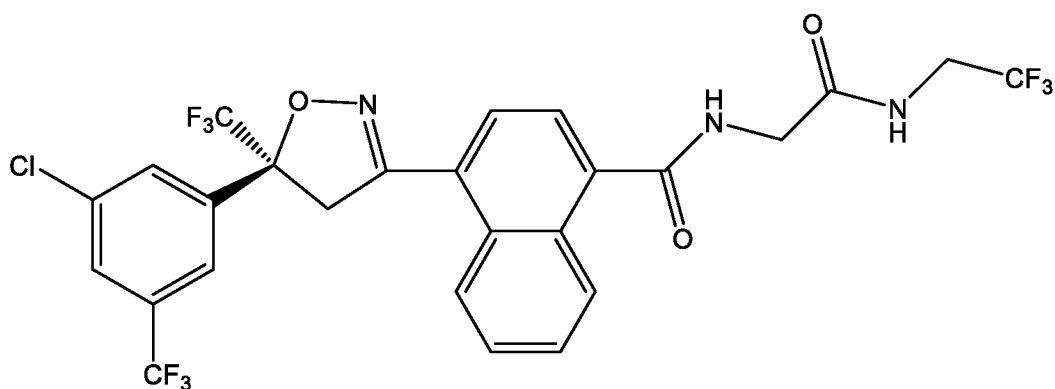
(S)-афоксоланер
