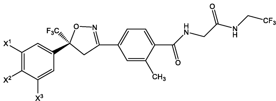
(S)-IB
