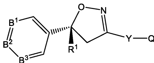
(R)-I
