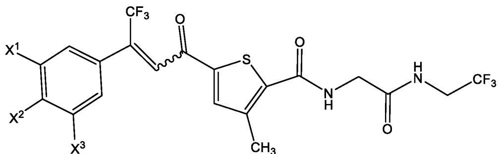
(IID)
