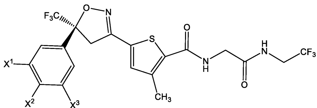
(S)-ID
