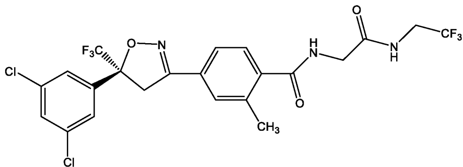
( S )-флураланер
