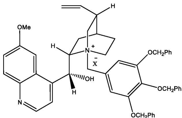
(Ша-13-1)
