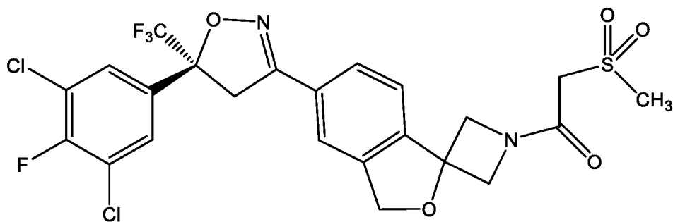
Сароланер
