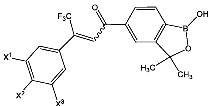
(IIA)
