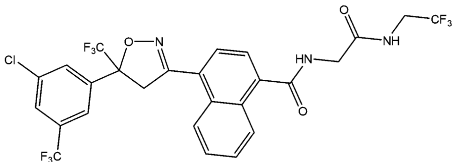
Афоксоланер
