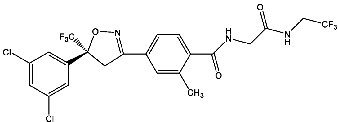
(S)-флураланер
