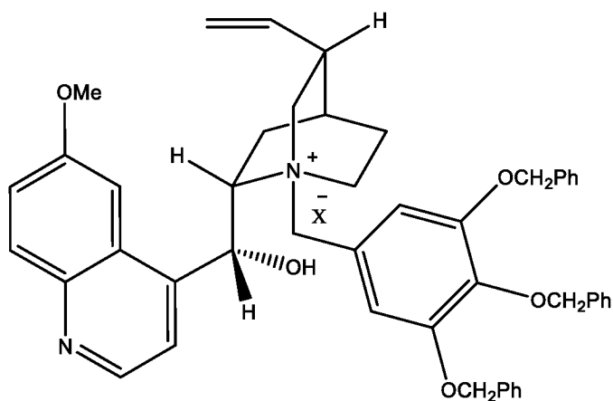
(Ша-13-1)
