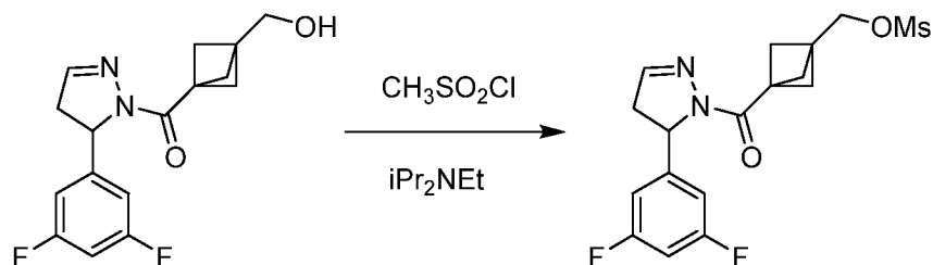
[0413] (3-(5-(3,5-Дифторфенил)-4,5-дигидро-1H-пиразол-1-карбонил)бицикло[1.1.1]пентан-1-ил)метила метансульфонат (промежуточное соединение II) К раствору продукта из предыдущей
