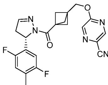
( S )-5-((3-(5-(2,5-Дифтор-4-метилфенил)-4,5-дигидро-1 H -пиразол-1-карбонил)бицикло[1.1.1]пентан-1-ил)метокси)пиразин-2-карбонитрил
