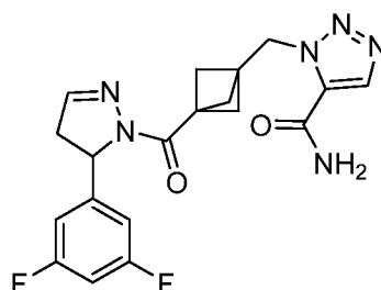
1-((3-(5-(3,5-Дифторфенил)-4,5-дигидро-1H-пиразол-1-карбонил)бицикло[1.1.1]пентан-1-ил)метил)-1H-1,2,3-триазол-5-карбоксамид
