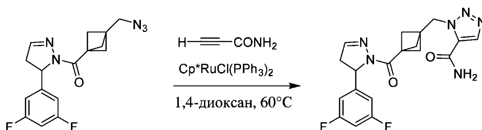
1-((3-(5-(3,5-Дифторфенил)-4,5-дигидро-1H-пиразол-1-карбонил)бицикло[1.1.1]пентан-1-ил)метил)-1H-1,2,3-триазол-5-карбоксамид
