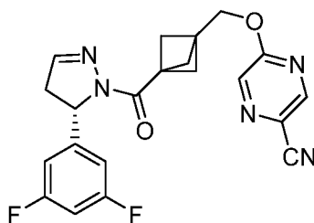
(S)-5-((3-(5-(3,5-Дифторфенил)-4,5-дигидро-1H-пиразол-1-карбонил)бицикло[1.1.1]пентан-1-ил)метокси)пиразин-2-карбонитрил
