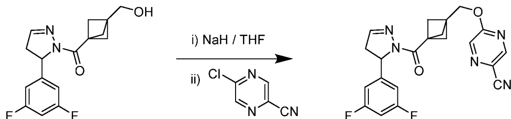
5-((3-(5-(3,5-Дифторфенил)-4,5-дигидро-1H-пиразол-1-карбонил)бицикло[1.1.1]пентан-1-ил)метокси)пиразин-2-карбонитрил
