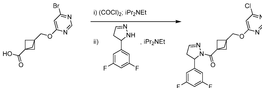
(3-(((6-Хлорпиримидин-4-ил)окси)метил)бицикло[1.1.1]пентан-1-ил)(5-(3,5-дифторфенил)-4,5-дигидро-1H-пиразол-1-ил)метанон
