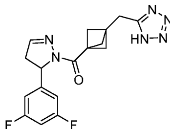
(3-((1H-Тетразол-5-ил)метил)бицикло[1.1.1]пентан-1-ил)(5-(3,5-дифторфенил)-4,5-дигидро-1H-пиразол-1-ил)метанон
