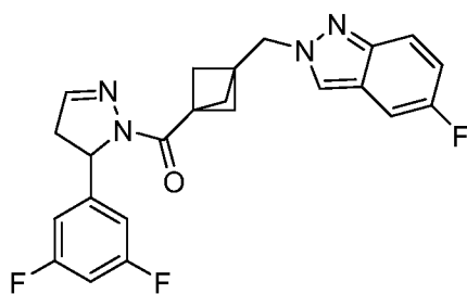
(5-(3,5-Дифторфенил)-4,5-дигидро-1H-пиразол-1-ил)(3-((5-фтор-2H-индазол-2-ил)метил)бицикло[1.1.1]пентан-1-ил)метанон (3)
