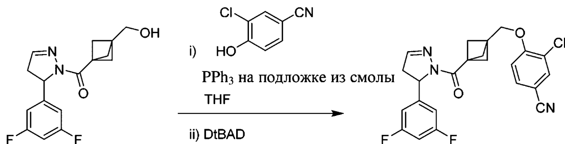
3-Хлор-4-((3-(5-(3,5-дифторфенил)-4,5-дигидро-1H-пиразол-1-карбонил)бицикло[1.1.1]пентан-1-ил)метокси)бензонитрил
