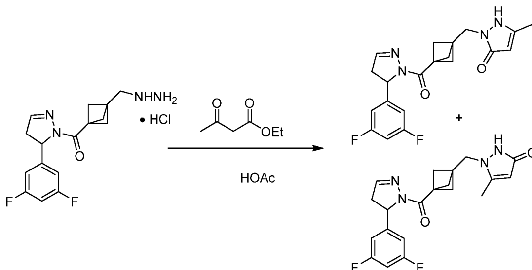
1-((3-(5-(3,5-дифторфенил)-4,5-дигидро-1H-пиразол-1-карбонил)бицикло[1.1.1]пентан-1-ил)метил)-5-метил-1,2-дигидро-3H-пиразол-3-он (16b)
