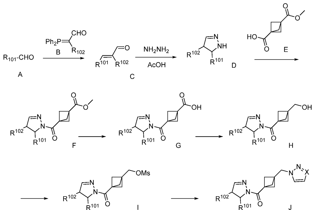
Схема I
