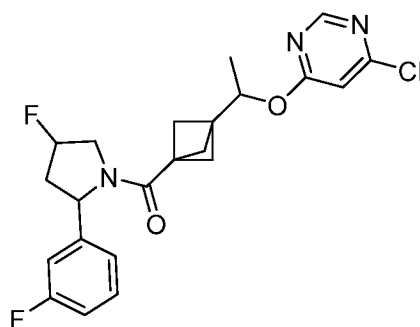
(3-(1-((6-Хлорпиримидин-4-ил)окси)этил)бицикло[1.1.1]пентан-1-ил)(4-фтор-2-(3-фторфенил)пирролидин-1-ил)метанон
