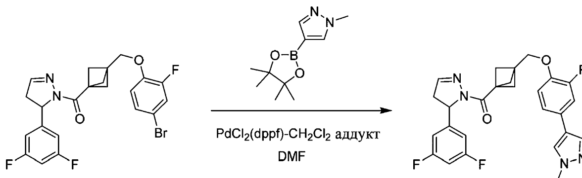
(5-(3,5-Дифторфенил)-4,5-дигидро-1Н-пиразол-1-ил)(3-((2-фтор-4-(1-метил-1Н-пиразол-4-ил)фенокси)метил)бицикло[1.1.1]пентан-1-ил)метанон
