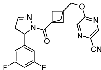
5-((3-(5-(3,5-Дифторфенил)-4,5-дигидро-1H-пиразол-1-карбонил)бицикло[1.1.1]пентан-1-ил)метокси)пиразин-2-карбонитрил
