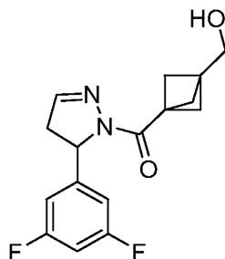
(5-(3,5-Дифторфенил)-4,5-дигидро-1H-пиразол-1-ил)(3-(гидроксиметил)бицикло[1.1.1]пентан-1-ил)метанон
