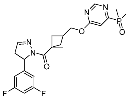
(5-(3,5-Дифторфенил)-4,5-дигидро-1H-пиразол-1-ил)(3-(((6-(диметилфосфорил)пиримидин-4-ил)окси)метил)бицикло[1.1.1]пентан-1-ил)метанон
