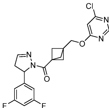
(3-(((6-Хлорпиримидин-4-ил)окси)метил)бицикло[1.1.1]пентан-1-ил)(5-(3,5-дифторфенил)-4,5-дигидро-1H-пиразол-1-ил)метанон
