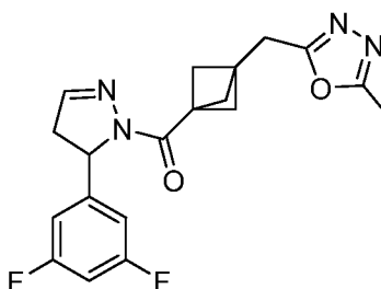
(5-(3,5-Дифторфенил)-4,5-дигидро-1H-пиразол-1-ил)(3-((5-метил-1,3,4-оксадиазол-2-ил)метил)бицикло[1.1.1]пентан-1-ил)метанон
