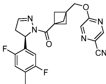
( R )-5-((3-(5-(2,5-Дифтор-4-метилфенил)-4,5-дигидро-1 H -пиразол-1-карбонил)бицикло[1.1.1]пентан-1-ил)метокси)пиразин-2-карбонитрил
