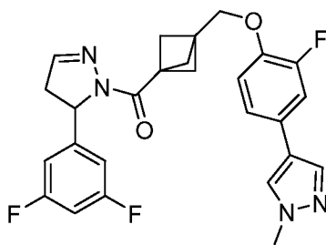
(5-(3,5-Дифторфенил)-4,5-дигидро-1Н-пиразол-1-ил)(3-((2-фтор-4-(1-метил-1Н-пиразол-4-ил)фенокси)метил)бицикло[1.1.1]пентан-1-ил)метанон
