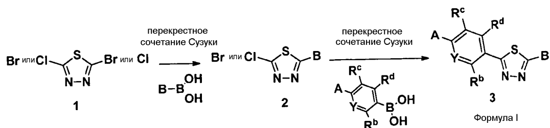
Общая схема 2
