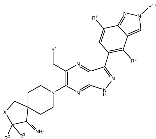
(VIIIa)
