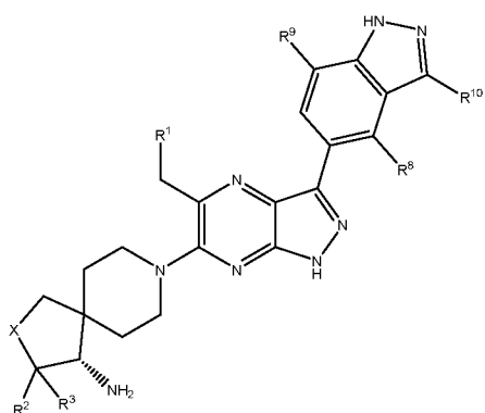
Таутомер А
