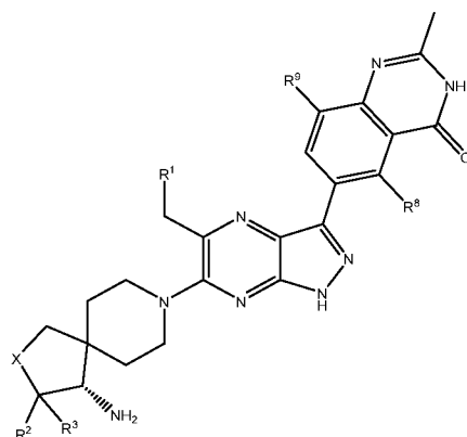
Таутомер В
