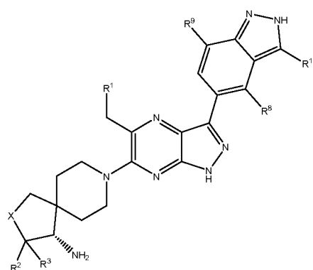
Таутомер В
