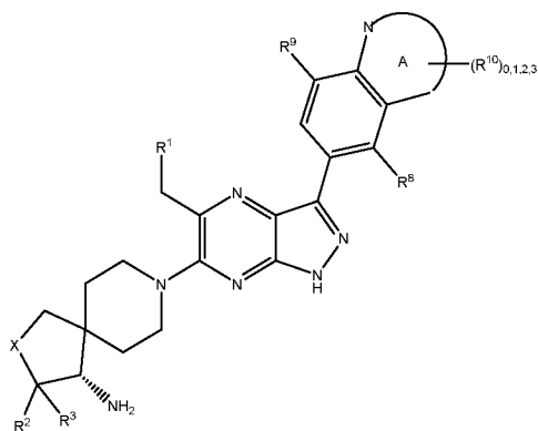
(XIIIa) или
