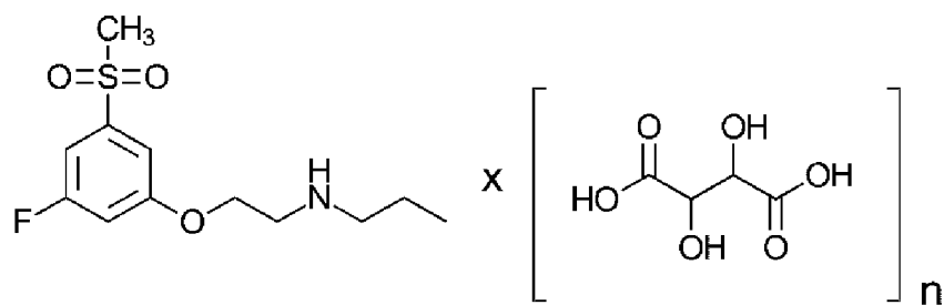
Формула IV
