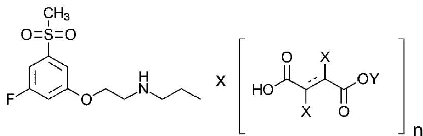
Формула III
