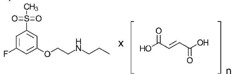
Формула V
