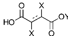
Формула II
