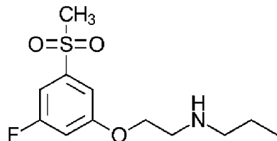
Формула I
