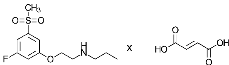
Формула Vb
