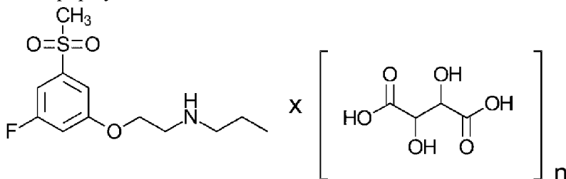
Формула IV.
