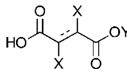
Формула II
