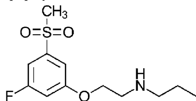
Формула I
