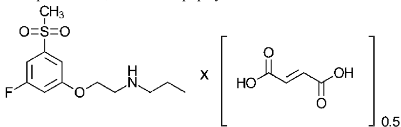
Формула Va
