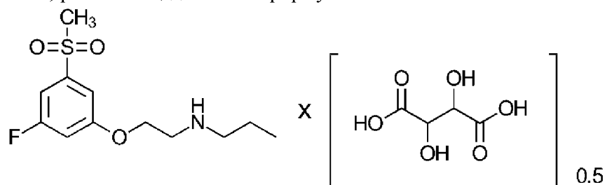
Формула IVa
