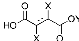
Формула II
