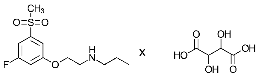
Формула IVb
