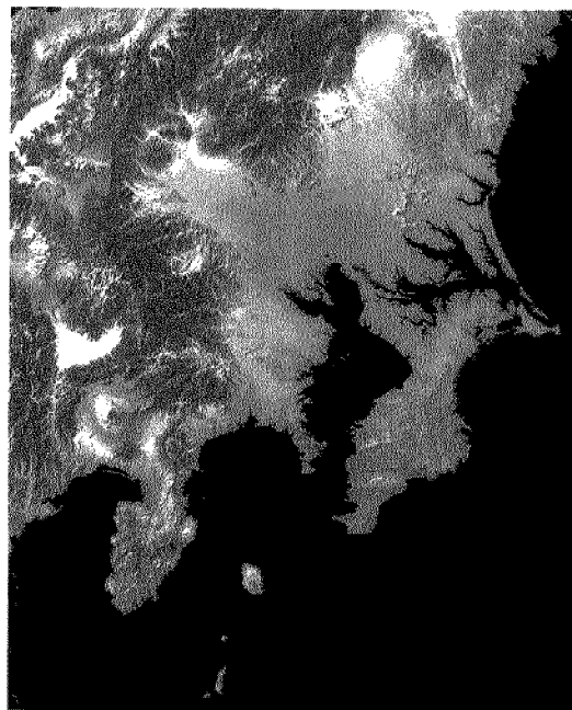
ОБЛАСТЬ КАНТО, ПЕРВАЯ ПОЛОВИНА ЭРЫ ДЗЕМОН (УРОВЕНЬ МОРЯ ПОДНЯТ, ПРИБЛИЗИТЕЛЬНО НА 5 м)
