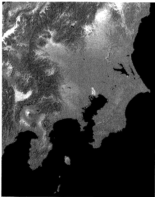
СЕГОДНЯШНЯЯ ОБЛАСТЬ КАНТО
