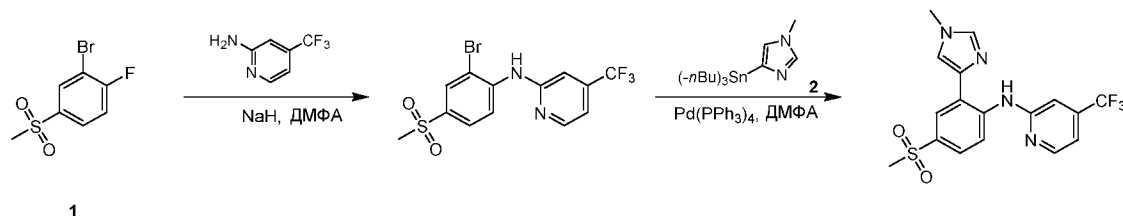
Стадия 1: N -(2-Бром-4-метилсульфонилфенил)-4-(трифторметил)пиридин-2-амин
