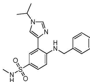
Стадия 1: 4-(Бензиламино)-3-(1-изопропилимидазол-4-ил)- N -метилбензолсульфонамид
