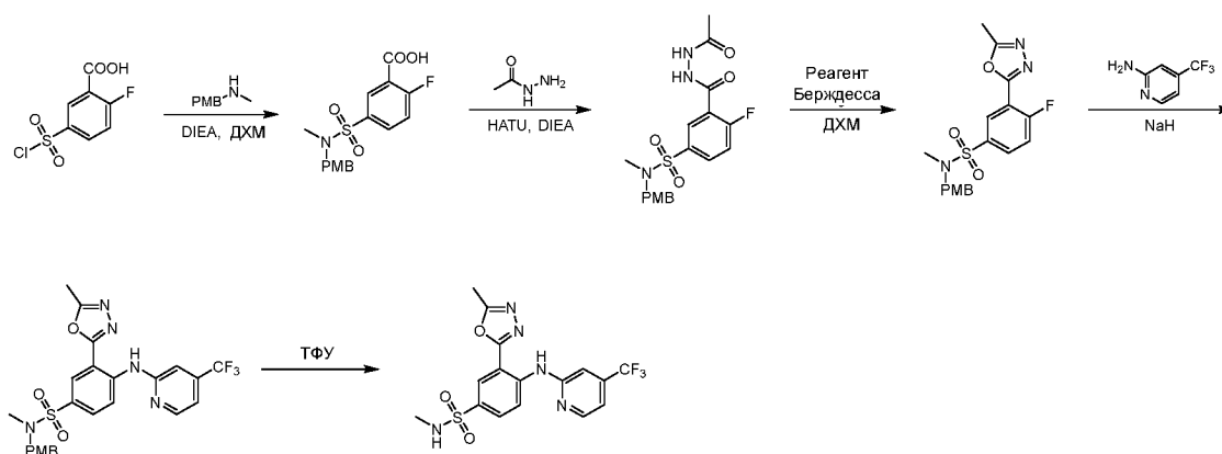
Стадия 1: 2-Фтор-5-[(4-метоксифенил)метил-метил-сульфамоил]бензойная кислота
