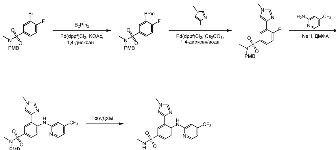
Стадия 1: 4-Фтор- N -[(4-метоксифенил)метил]- N -метил-3-(4,4,5,5-тетраметил-1,3,2-диоксаборолан-2-ил)бензолсульфонамид
