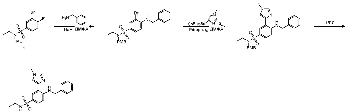
Стадия 1: 4-(Бензиламино)-3-бром-N-этил-N-[(4-метоксифенил)метил]бензолсульфонамид
