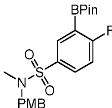
Стадия 1: 4-Фтор- N -[(4-метоксифенил)метил]- N -метил-3-(4,4,5,5-тетраметил-1,3,2-диоксаборолан-2-ил)бензолсульфонамид
