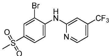
Стадия 1: N -(2-Бром-4-метилсульфонилфенил)-4-(трифторметил)пиридин-2-амин
