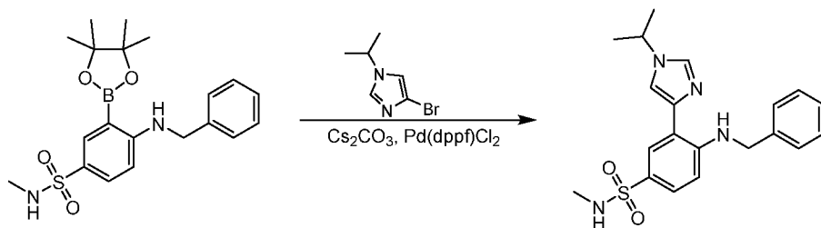
Стадия 1: 4-(Бензиламино)-3-(1-изопропилимидазол-4-ил)- N -метилбензолсульфонамид
