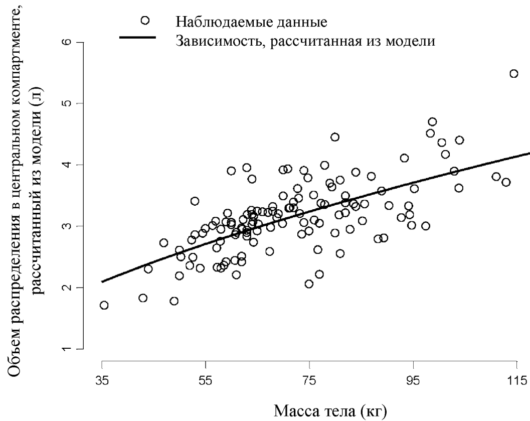
Фиг. 4. Зависимость объема распределения в центральном компартменте, рассчитанного из популяционной фармакокинетической модели, от массы тела в исследовании из примера 1.
