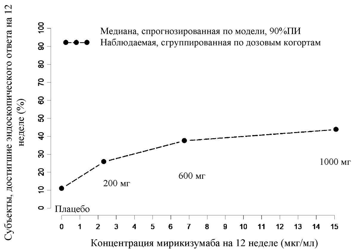
Фиг. 5. Визуальная оценка предсказательной способности подбора модели для эндоскопического ответа на 12 неделе в исследовании из примера 1.
