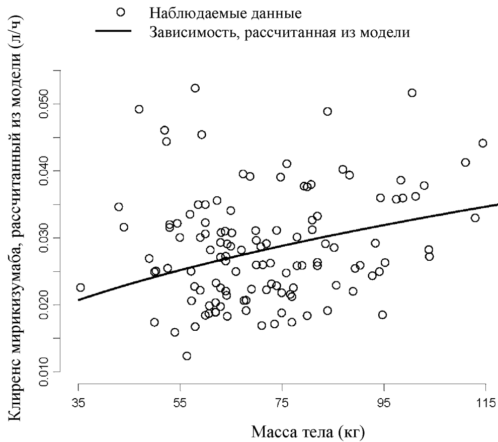
Фиг. 3. Зависимость клиренса, рассчитанного из популяционной фармакокинетической модели, от массы тела в исследовании из примера 1.
