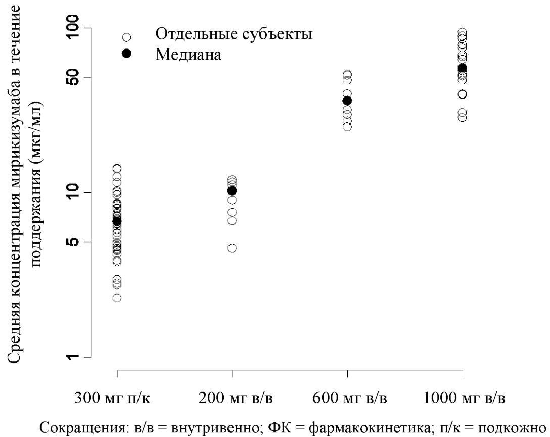
Фиг. 2. Средние сывороточные концентрации мирикизумаба в течение поддерживающего периода в исследовании, описанном в примере 1.
