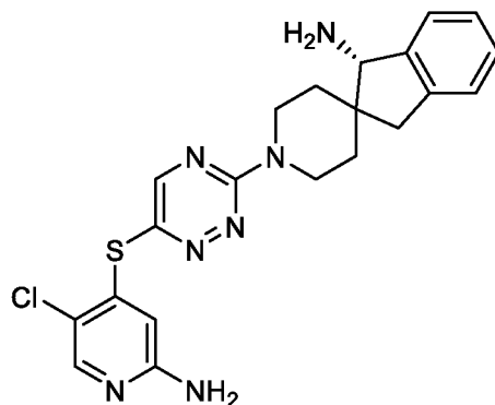
( S )-1'-(6-((2-амино-5-хлорпиридин-4-ил)тио)-1,2,4-триазин-3-ил)-1,3-дигидроспиро[инден-2,4'-пиперидин]-1-амин
