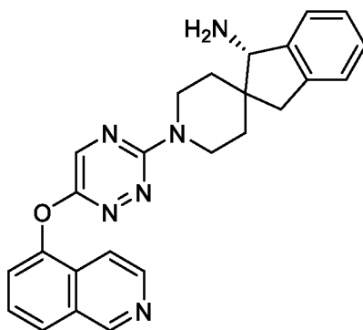
( S )-1'--(6-(изохинолин-5-илокси)-1,2,4-триазин-3-ил)-1,3-дигидроspиро[инден-2,4'-пиперидин]-1-амин
