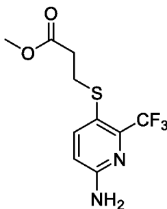
метил 3-((6-амино-2-(трифторметил)пиридин-3-ил)тио)пропаноат
