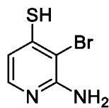
2-амино-3-бромпиридин-4-тиол
