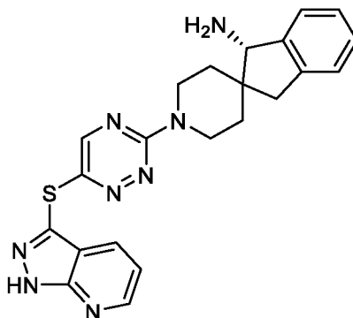
( S )-1'--(6-((1 H -пирразоло[3,4- b ]пиридин-3-ил)тио)-1,2,4-триазин-3-ил)-1,3-дигидроspиро[инден-2,4'-пиперидин]-1-амин
