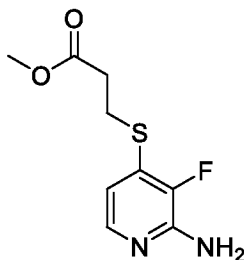
метил 3-((2-амино-3-фторпиридин-4-ил)тио)пропаноат
