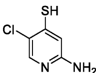
2-амино-5-хлорпиридин-4-тиол
