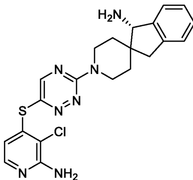
( S )-1'-((2-амино-3-хлорпиридин-4-ил)тио)-1,2,4-триазин-3-ил)-1,3-дигидроспиро[инден-2,4'-пиперидин]-1-амин
