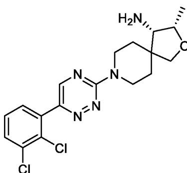
(3 S ,4 S )-8-(6-(2,3-дихлорфенил)-1,2,4-триазин-3-ил)-3-метил-2-окса-8-азаспиро[4.5]декан-4-амин
