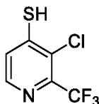
3-хлор-2-(трифторметил)пиридин-4-тиол
