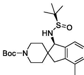
tert-бутил (R)-1-(((R)-tert-бутилсульфинил)амино)-4-метил-1,3- дигидроспиро[инден-2,4'-пиперидин]-1'-карбоксилат
