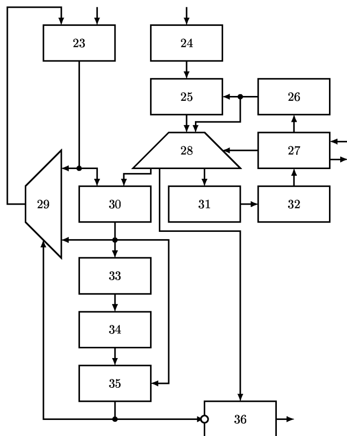
Фиг. 3. Блок уточнения аппроксимационного ряда
