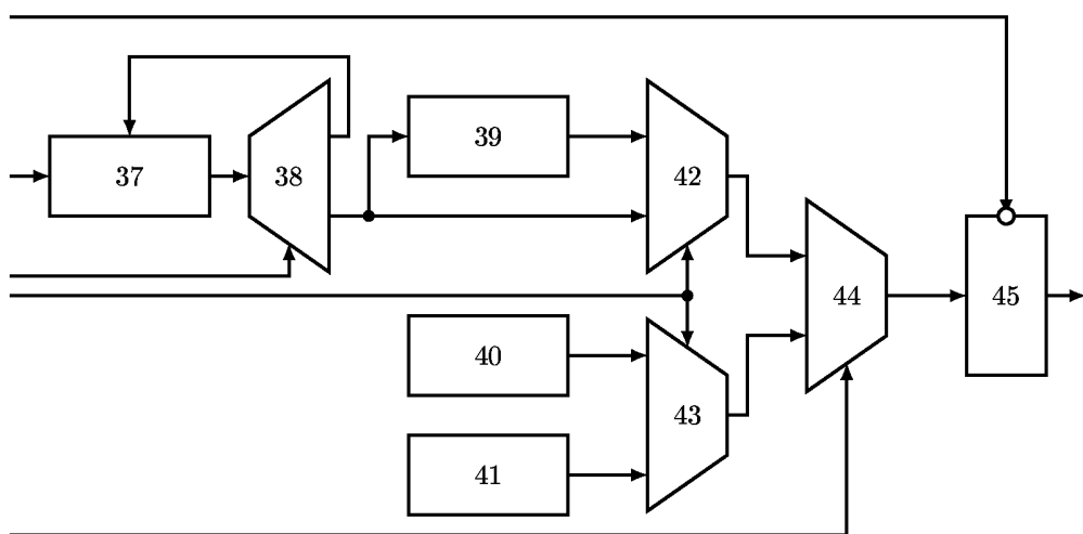
Фиг. 4. Блок вывода частного
