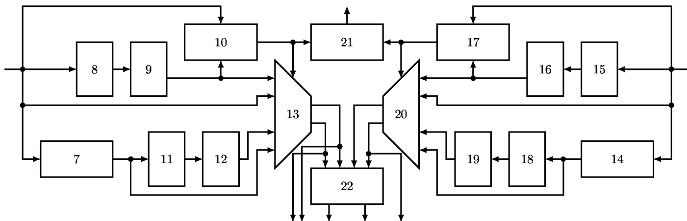
Фиг. 2. Блок вычисления позиционных характеристик
