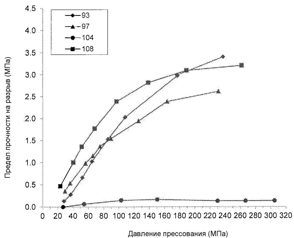
Графики зависимости предела прочности на разрыв компактов от давления прессования
