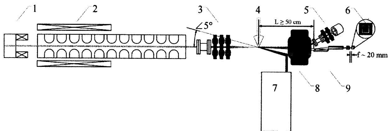
Рисунок 1. Общий вид установки: 1 – электронная пушка; 2 – линейный ускоритель электронов; 3 – система фокусировки электронного пучка; 4 – точка столкновения электронного и фотонного пучков; 5 – электронная ловушка; 6 – испытуемый образец; 7 – лазерная система; 8 – отклоняющий магнит; 9 – рентгеновская оптика.
