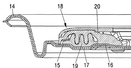
Фрагмент В Фиг. 8
