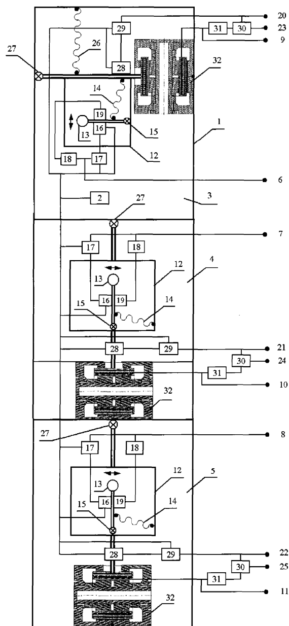
Трехкомпонентный скважинный сейсмометр
