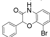
Стадия 1. 8-Бром-2-фенил-2Н-1,4-бензоксазин-3(4Н)-он.
