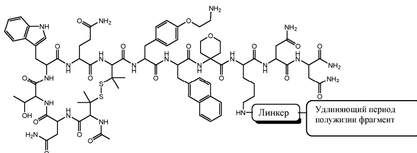
Пример 10. Ac-[Pen]-NTWQ-[Pen]-[Phe[4-(аминоэтокси)]-[2-Nal]-[4-амино-4-карбокситетрагидропиран]-[Lys(линкер-удлиняющий период полужизни фрагмент)]-NN-NH 2 (SEQ ID NO: 1478).
