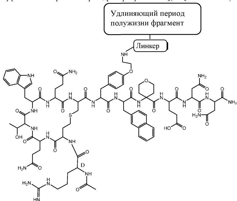
Пример 3а. Ас-[(D)-Arg]цикло[[Abu]-QTWQC]-[Phe[4-(2-аминоэтокси)-(линкер-удлиняющий период полужизни фрагмент)]-[2-Nal]-[4-амино-4-карбокситетрагидропиран]-ENN-NH 2 (SEQ ID NO: 1468)
