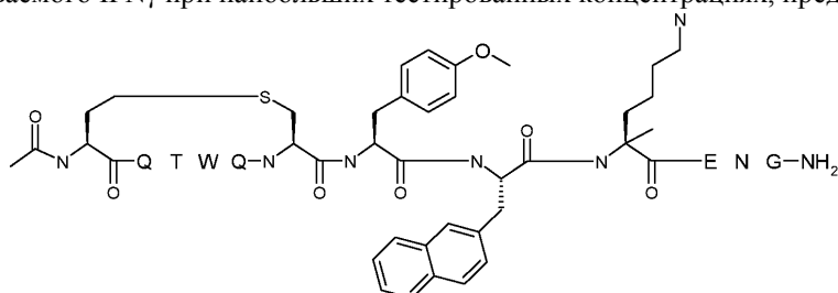
Соединение А (SEQ ID NO: 258)
