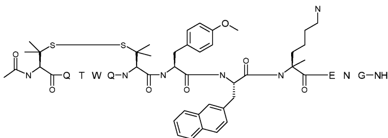
Соединение В (SEQ ID NO: 282)
