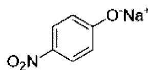
натрия п-нитрофенолат
