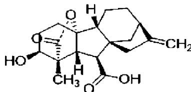
гиббереллин A 4
