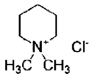
мепиквата хлорид
