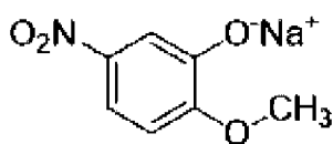
натрия 5-нитрогуаиаколат
