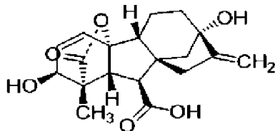
гибберелинновая кислота
