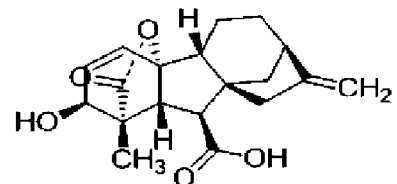
гиббереллин A 7
