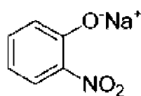
натрия о-нитрофенолат
