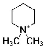
мепиквата пентаборат
