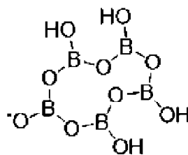
мепиквата пентаборат
