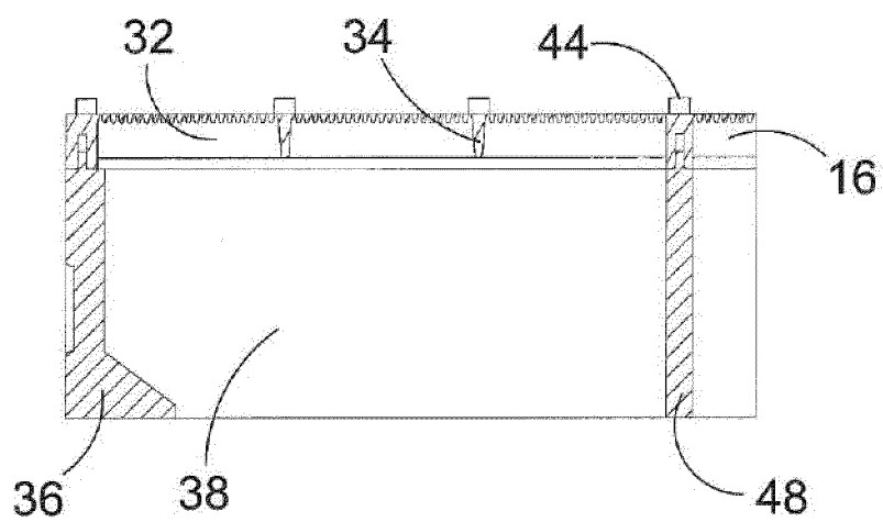
Разрез В-В
