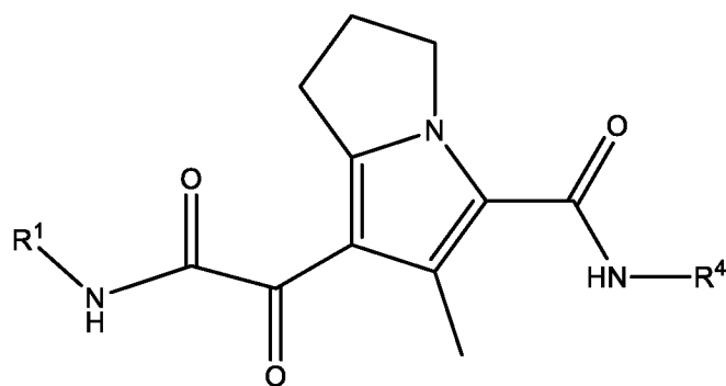
Формула IV
