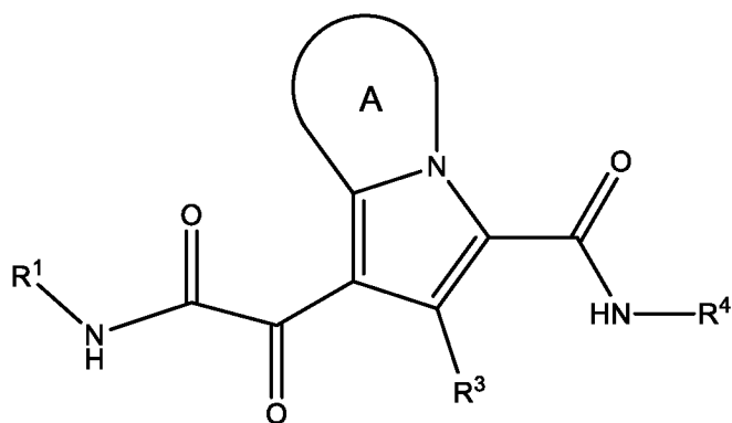
Формула I
