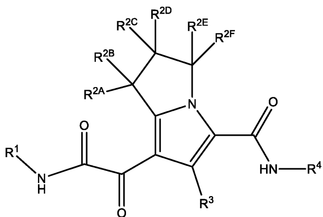
Формула II
