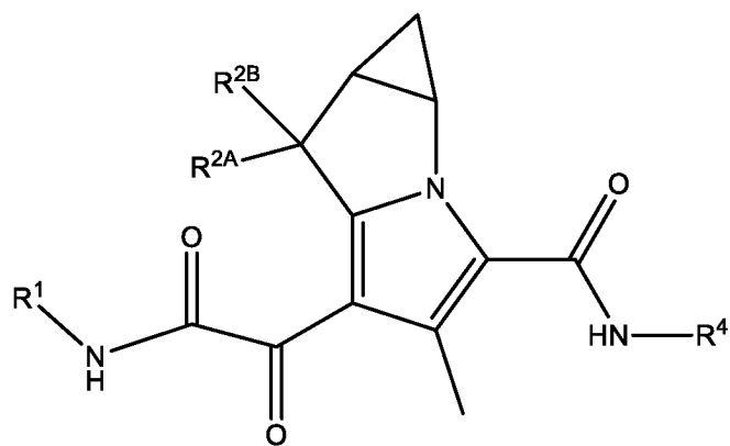
Формула III
