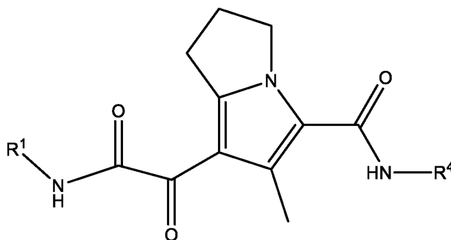
Формула IV
