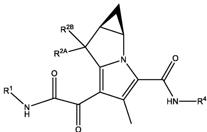
Формула IIIa
