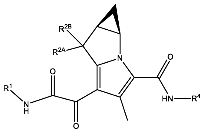
Формула IIIa
