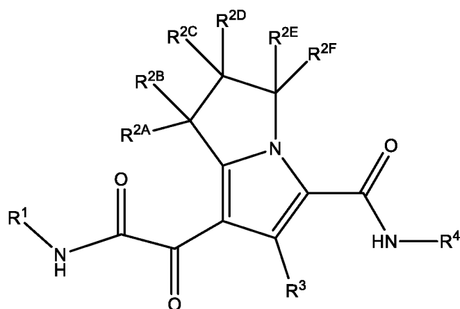
Формула II
