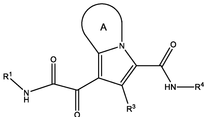
Формула I
