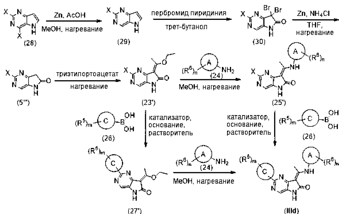
Схема синтеза 3
