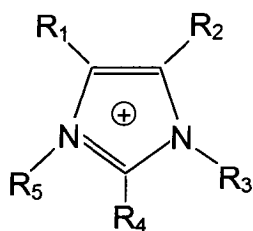
Имидазолий
