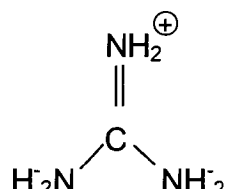
Гуанидиний
