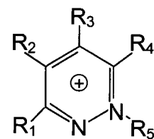
Пиридазиний
