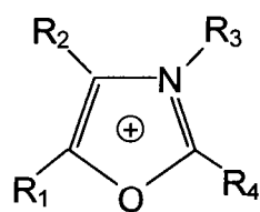
Оксазолий
