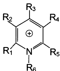
Пиридиний
