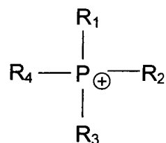
Фосфоний
