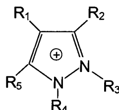
Пиразолий
