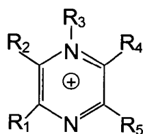
Пиразиний
