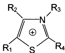
Тиазолий
