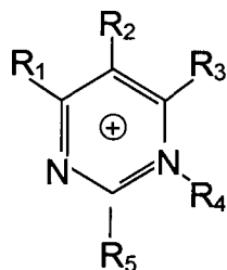
Пиримидиний
