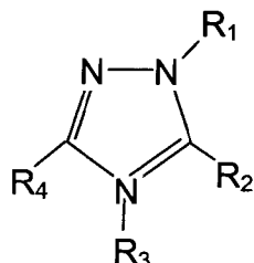
Триазолий
