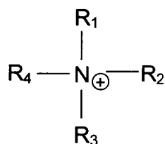
Аммоний
