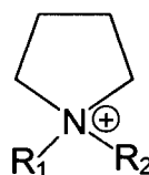
Пирролидиний
