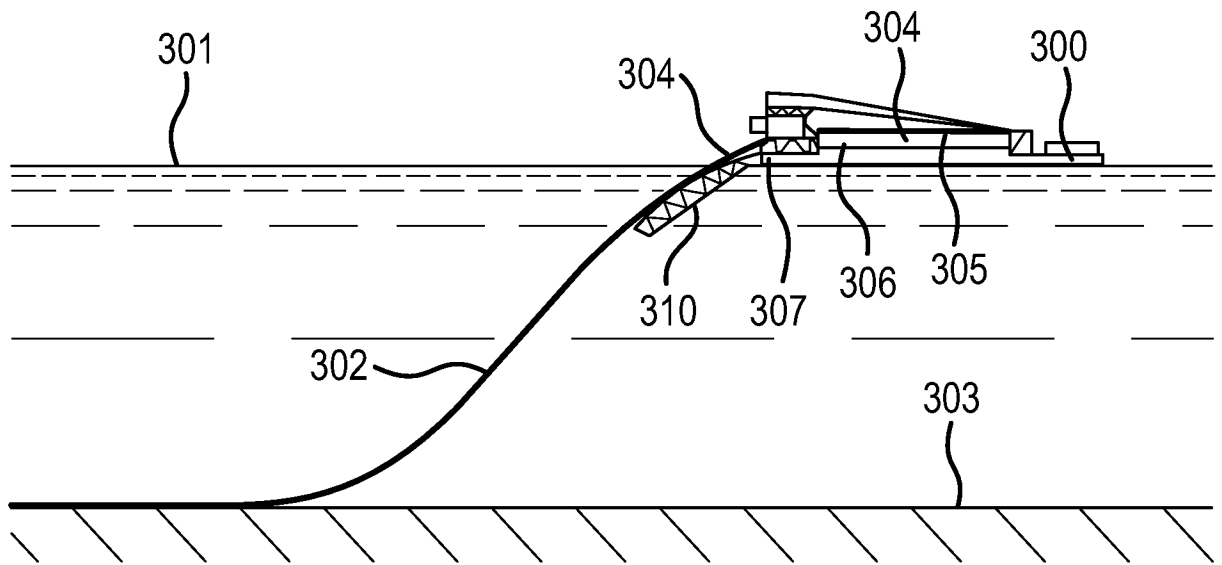
ФИГ. 14 (УРОВЕНЬ ТЕХНИКИ)
