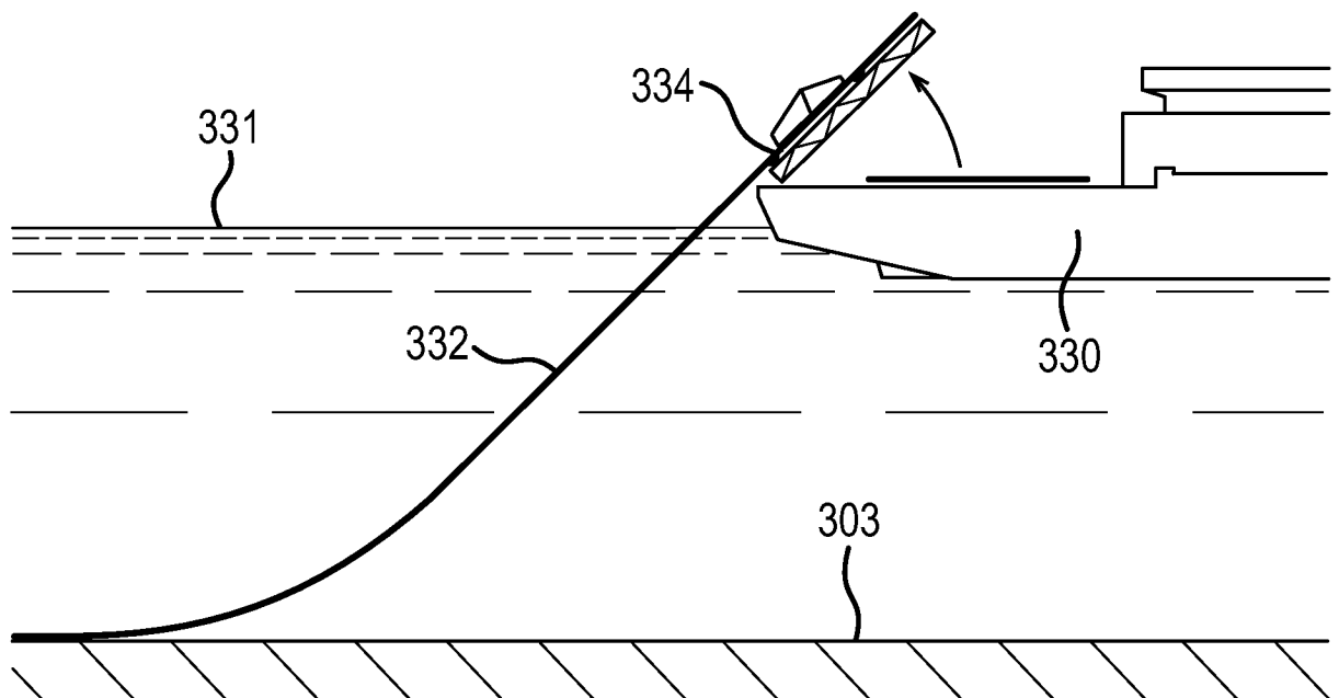
ФИГ. 15 (УРОВЕНЬ ТЕХНИКИ)
