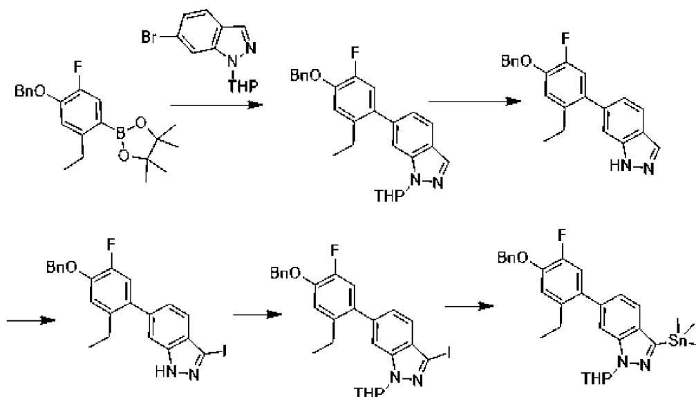
(а) 6-(4-(Бензилокси)-2-этил-5-фторфенил)-1-(тетрагидро-2Н-пиран-2-ил)-1Н-индазол
