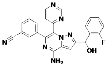
Пример 23. 3-(4-Амино-2-((2-фторфенил)(гидрокси)метил)-7-(пиримидин-4-ил)пиразоло[1,5-а]пиразин-6-ил)бензонитрил
