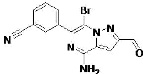
Стадия 1. 3-(4-Амино-7-бром-2-формилтиразоло[1,5-а]пиразин-6-ил)бензонитрил
