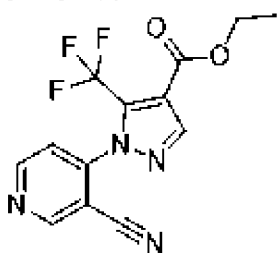
, соединение 46c
