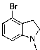
, соединение 128a
