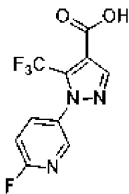
, соединение 121c
