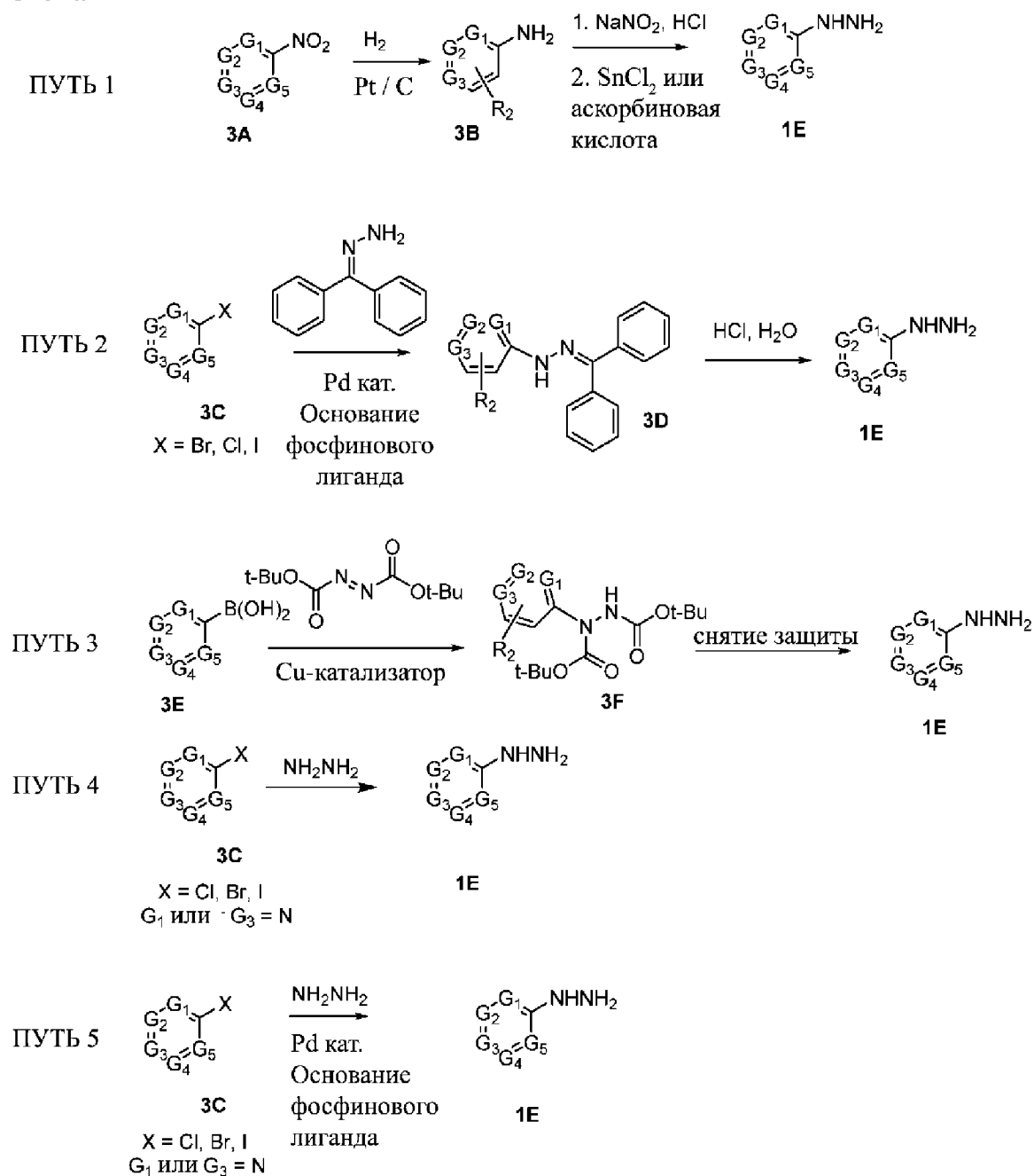
Схема 3
