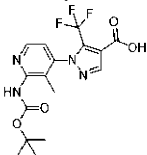
, соединение 143с
