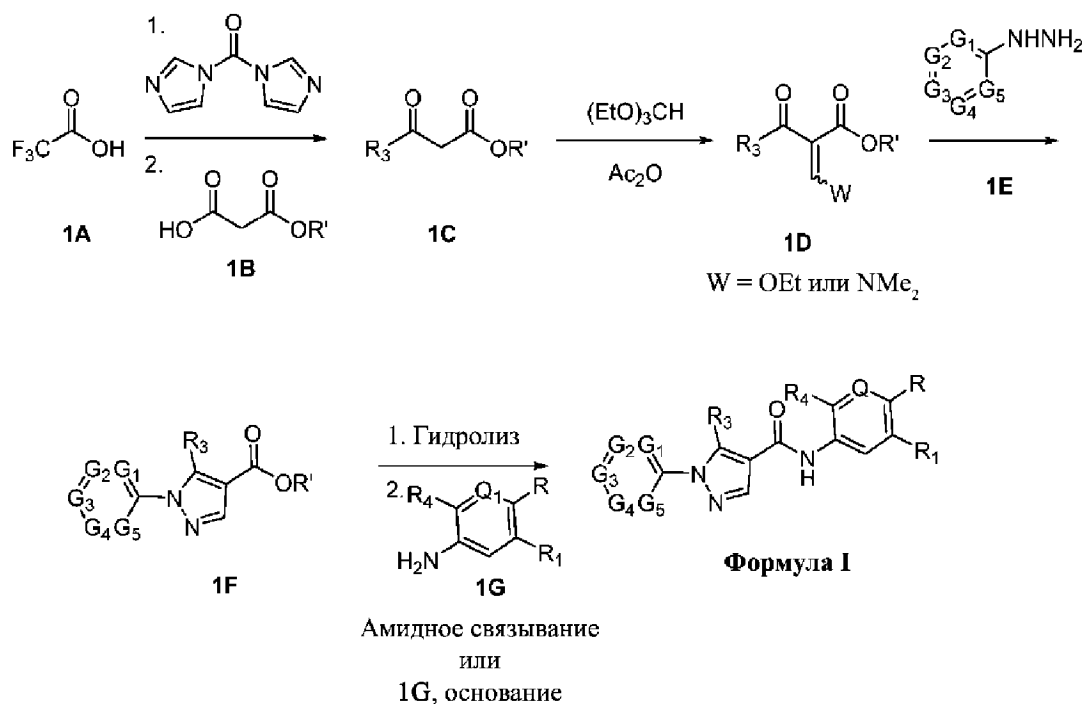
Схема 1
