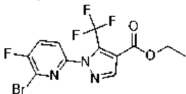
, соединение 151d
