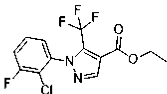
В. Этил 1-(2-хлор-3-фторфенил)-5-(трифторметил)-1Н-пиразол-4-карбоксилат, соединение 61b
