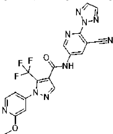
соединение 41
