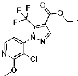
, соединение 32с
