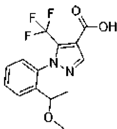
, соединение 118d
