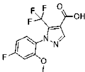
, соединение 54c
