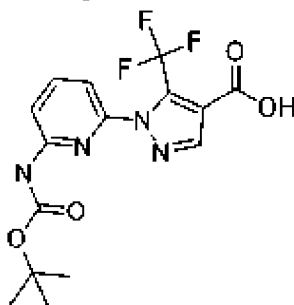
, соединение 134c
