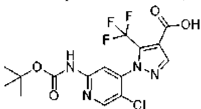
, соединение 148d
