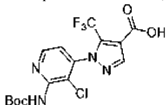
, соединение 56e
