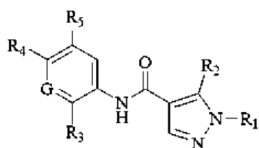
Формула (I)
