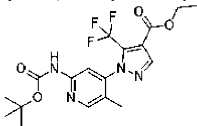
, соединение 142e
