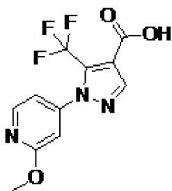
, соединение 41a
