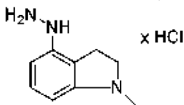
, соединение 128c
