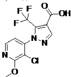
, соединение 32d
