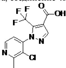
, соединение 43c
