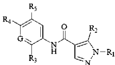
Формула (I)
