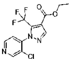
, соединение 45a
