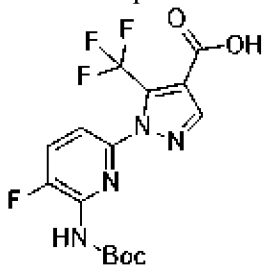
соединение 62d
