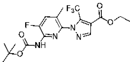
, соединение 145e
