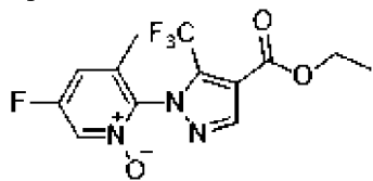
, соединение 145c
