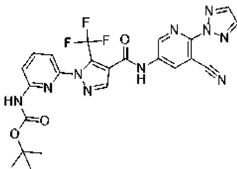
, соединение 134d
