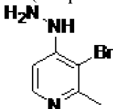
, соединение 33b
