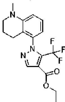
, соединение 127e
