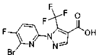
, соединение 151e
