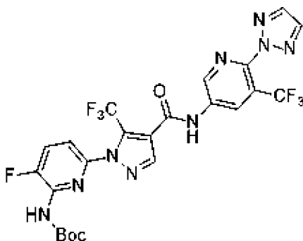
, соединение 147c
