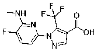
, соединение 150d
