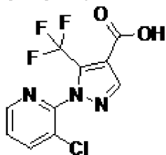
, соединение 44b
