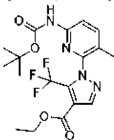
, соединение 141e
