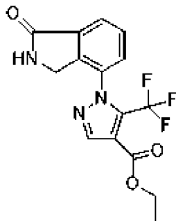
, соединение 133c
