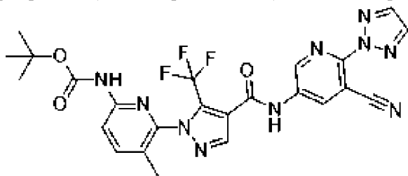
, соединение 141g
