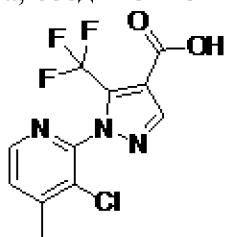
соединение 47с
