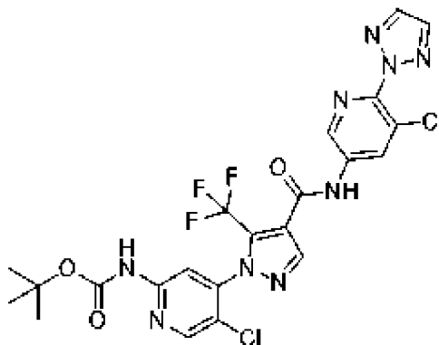
, соединение 149а
