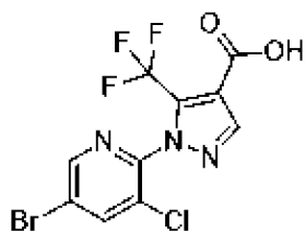
, соединение 30b
