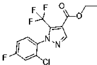
, соединение 51a
