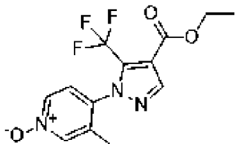
, соединение 142с
