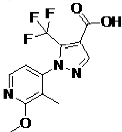
, соединение 38f
