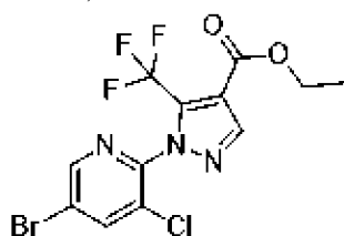
, соединение 30a
