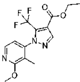
, соединение 38e
