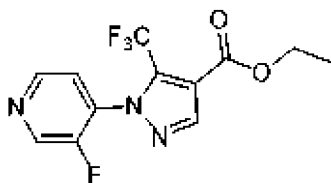
, соединение 6b
