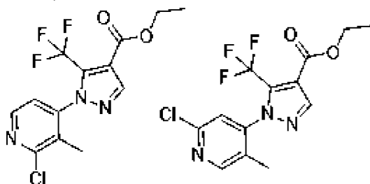
, соединение 142d
