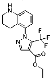
, соединение 127d
