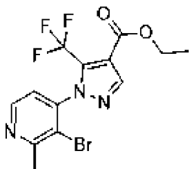
, соединение 33с
