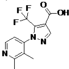
соединение 42с
