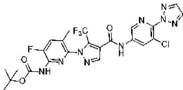
, соединение 146a
