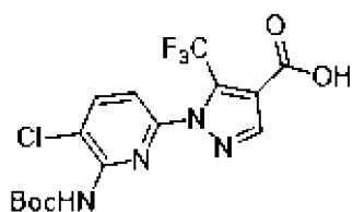
, соединение 144d
