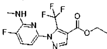
, соединение 150с
