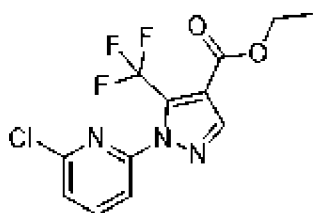
, соединение 44а
