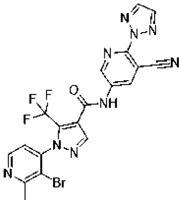
, соединение 33e
