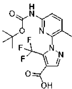
, соединение 141f
