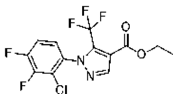
, соединение 60b
