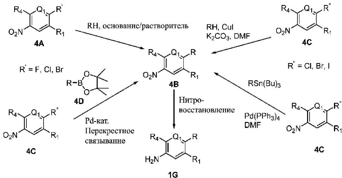
Схема 4
