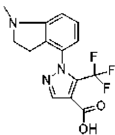
, соединение 128e
