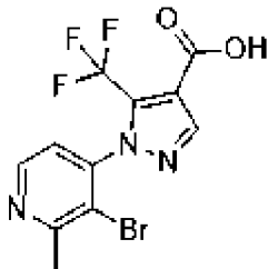
, соединение 33d
