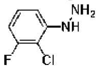
А. (2-Хлор-3-фторфенил)гидразин, соединение 61a
