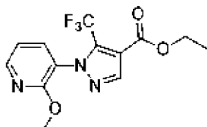
, соединение 14с
