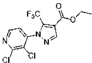
, соединение 56b
