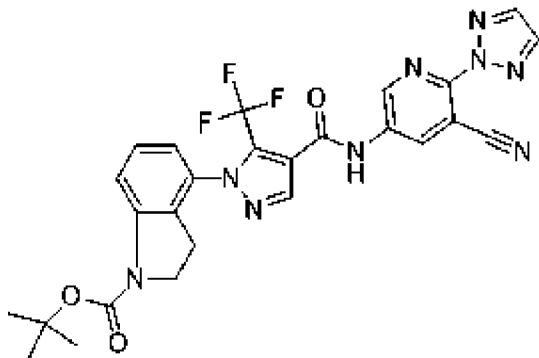
, соединение 130g
