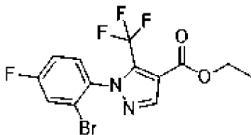
, соединение 50b
