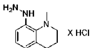
соединение 131c
