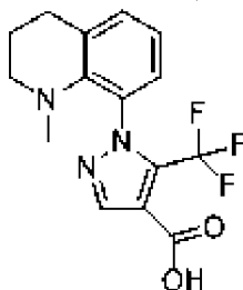
, соединение 131e
