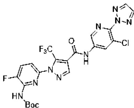
соединение 62e
