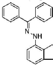
, соединение 128b
