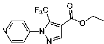
, соединение 4a
