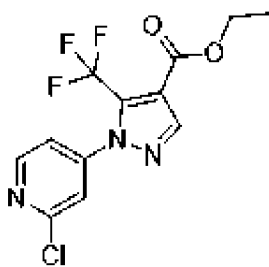
, соединение 39a
