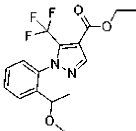
, соединение 118c
