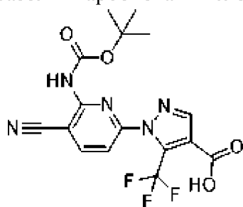
соединение 139d
