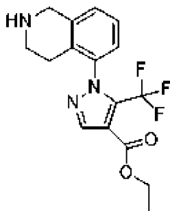
, соединение 129c
