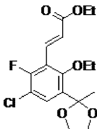
Стадия 2. Этил (2E)-3-[3-хлор-6-этокс-2-фтор-5-(2-метил-1,3-диоксолан-2-ил)фенил]акрилат
