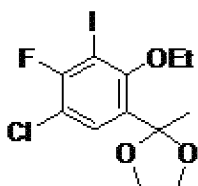
Стадия 1. 1-(5-Хлор-2-этокс-3-йод-4-метилфенил)этанол.
