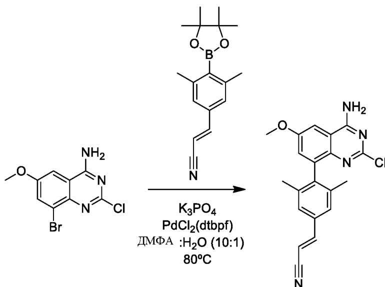
Соединение 24d
