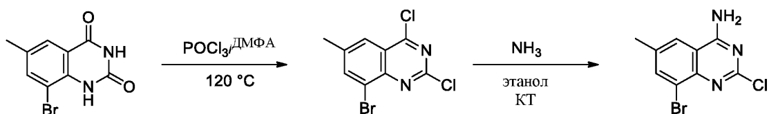
Соединение 21c
