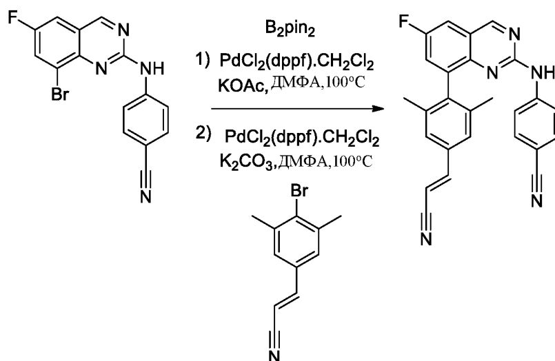
Соединение 4
