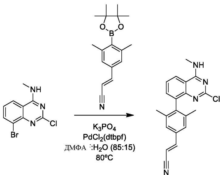
Соединение 30b
