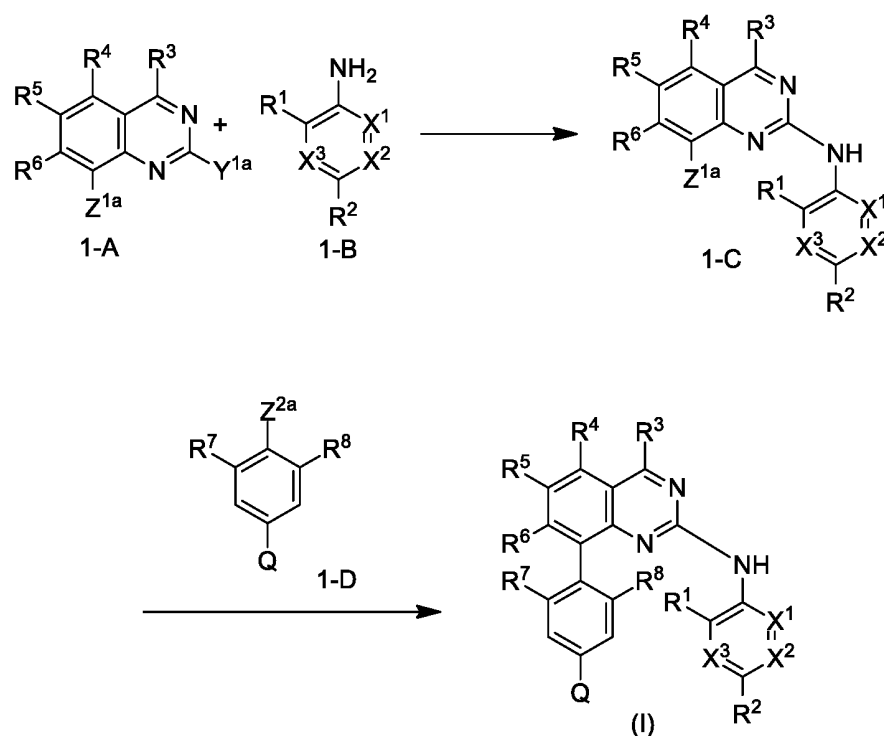
Схема 1
