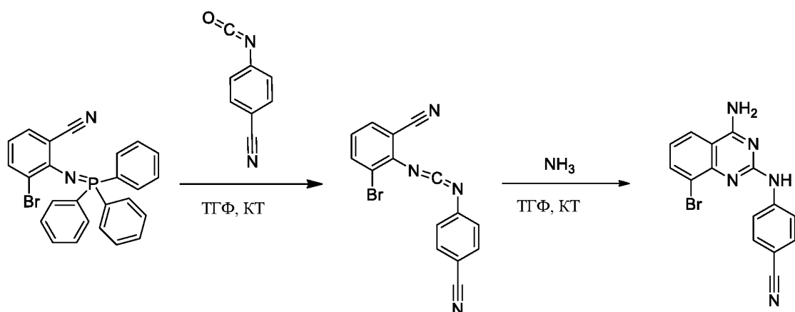
Соединение 8a
