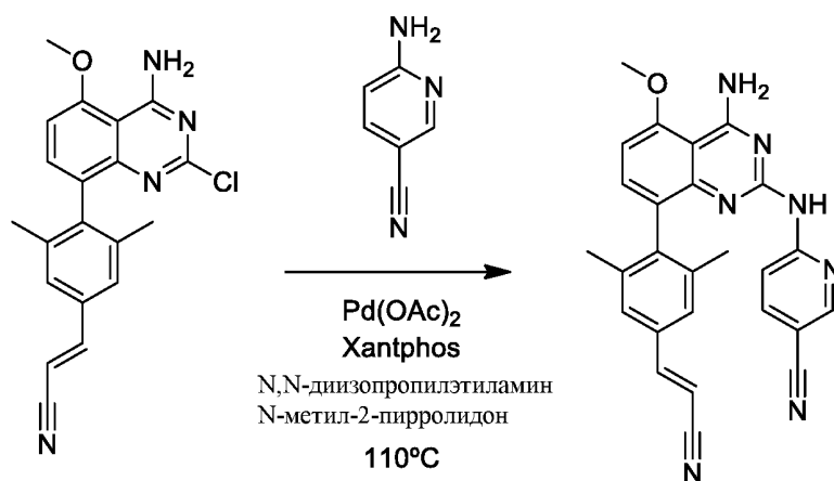
Соединение 29
