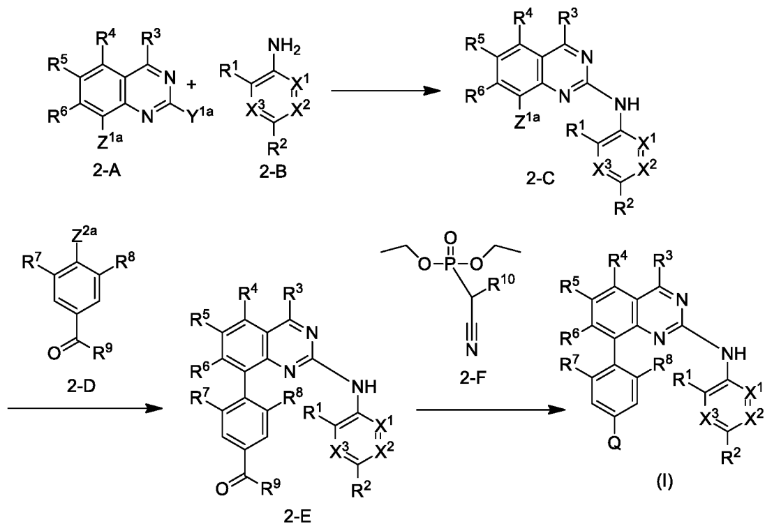
Схема 2
