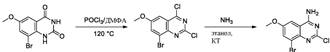
Соединение 24с
