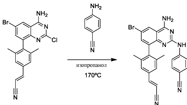
Соединение 25
