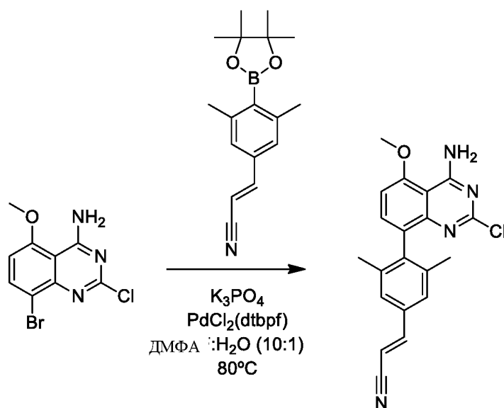
Соединение 28с
