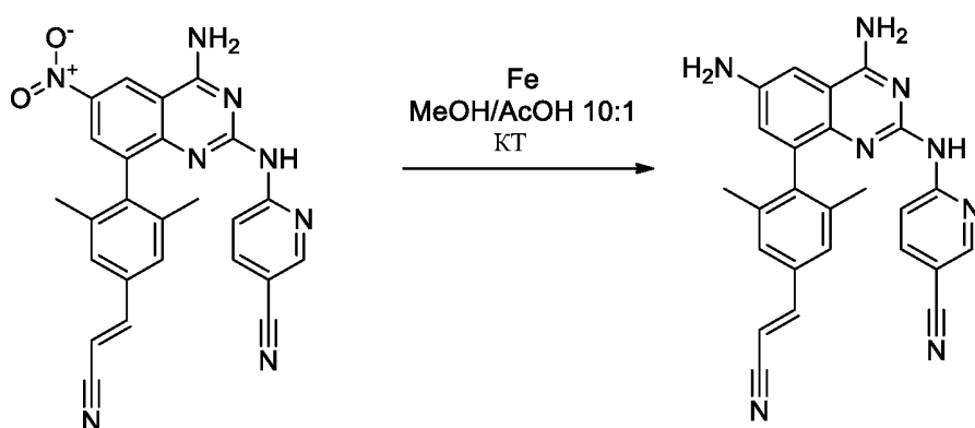
Соединение 23
