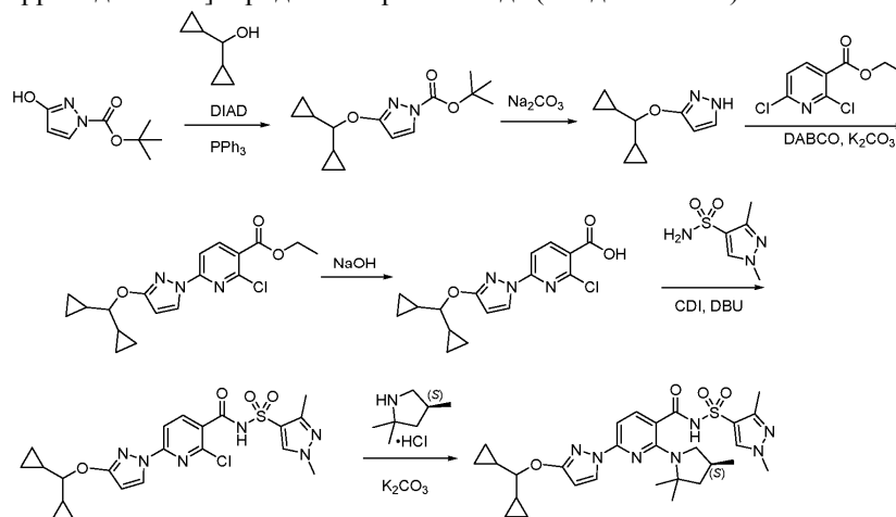
Стадия 1. трет-Бутил-3-(дициклопропилметокси)пиразол-1-карбоксилат
