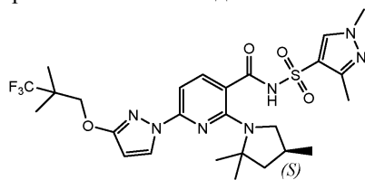
(Соединение 1);
