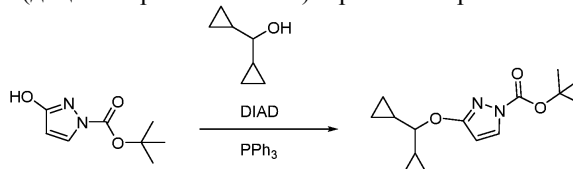
Стадия 1. трет-Бутил-3-(дициклопропилметокси)пиразол-1-карбоксилат
