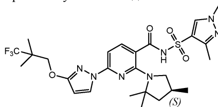
(Соединение 1);
