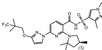
(Соединение 1);
