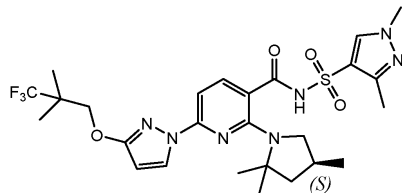
(Соединение 1);
