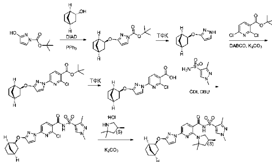
Стадия 1. трет-Бутил-3-(((1S,2S,4R)-бицикло[2.2.1]гептан-2-ил)окси)-1H-пиразол-1-карбоксилат
