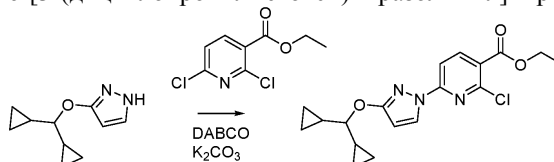
Стадия 3. Этил-2-хлор-6-[3-(дициклопропилметокси)пиразол-1-ил]пиридин-3-карбоксилат
