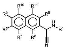
Формула (XLVu); и
