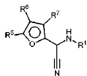
Формула (XLVg);
