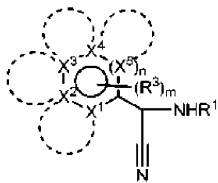
Формула (XLVb);
