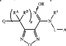
Формула (XVa); или
