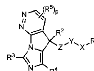
Формула (XLIXg);
