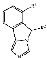
Формула (Xe);
