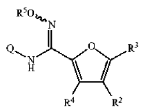
Формула (Vc); и
