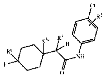
Формула (XLIIIq);
