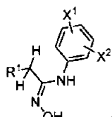
Формула (LVa);
