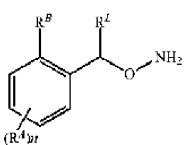
Формула (XXVIIIba); и
