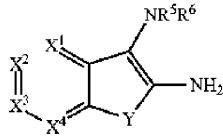
Формула (XXa);
