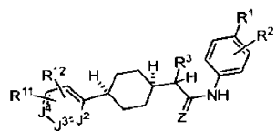
Формула (LIVo);
