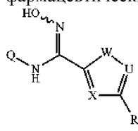
Формула (Va);
