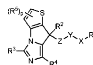
Формула (XLIXj).
