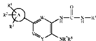
Формула (XXXIX); или
