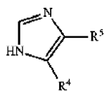
Формула (IXah);
