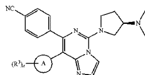
Формула (XVIIIo); и
