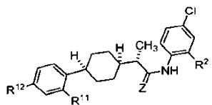
Формула (LIVz); и
