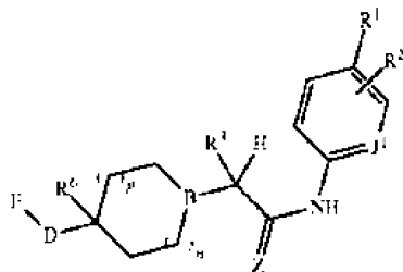
Формула (XLIIIg);
