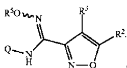
Формула (IVb); и
