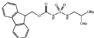
Формула F19; и
