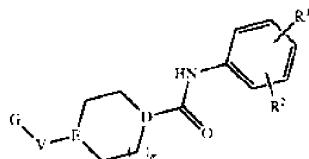
Формула (XLIVm); и
