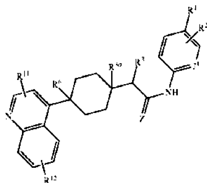
Формула (XLIIIm);
