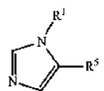
Формула (IXa);
