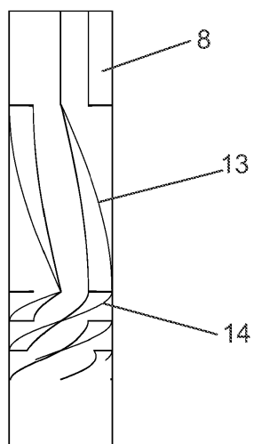
(разрез по линии В-В на фиг. 8) Фиг. 9
