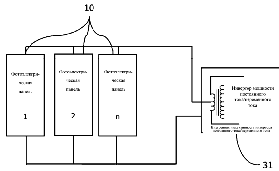
Фиг. 2А. Известный уровень техники
