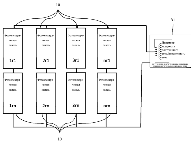
Фиг. 2С. Известный уровень техники
