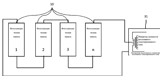
Фиг. 2В. Известный уровень техники
