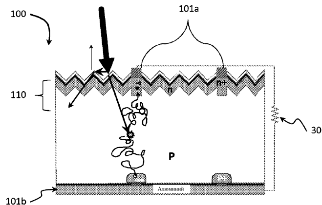
Фиг. 1. Известный уровень техники
