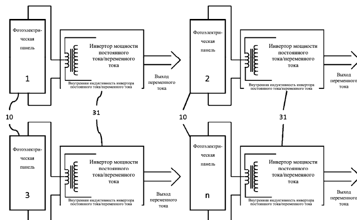
Фиг. 2D. Известный уровень техники
