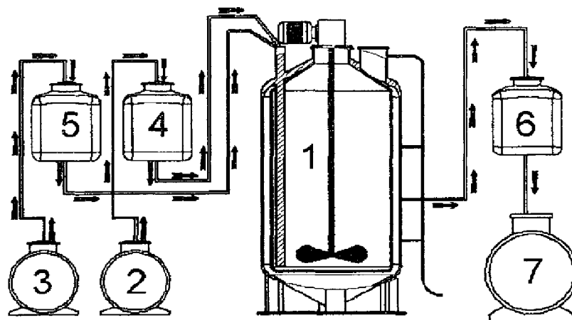
Фиг. 1. Технологическая схема производства полиметиламинового поверхностно-активного вещества
