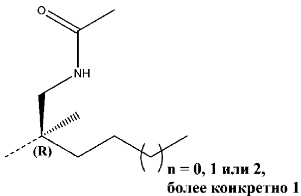
формула (V)
