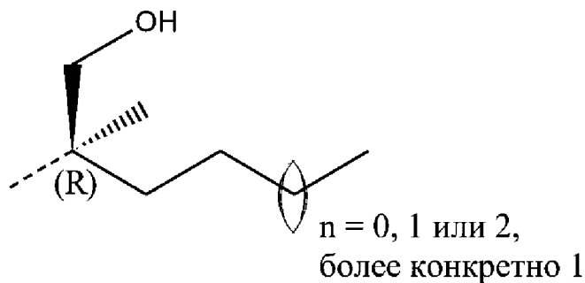
формула (III)
