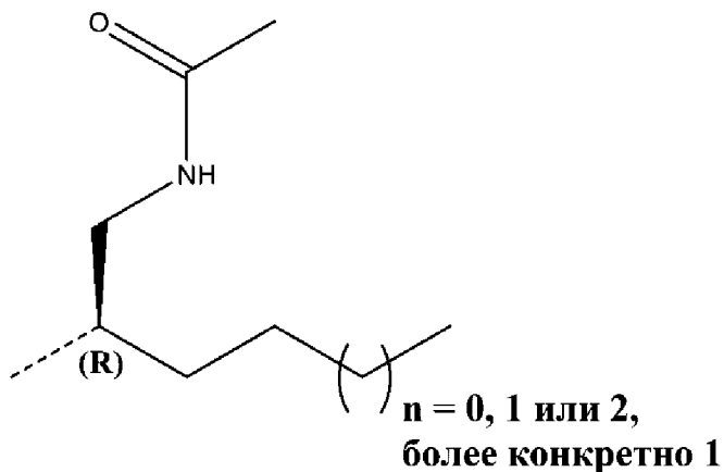
формула (IV)
