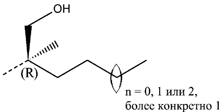
формула (III)
