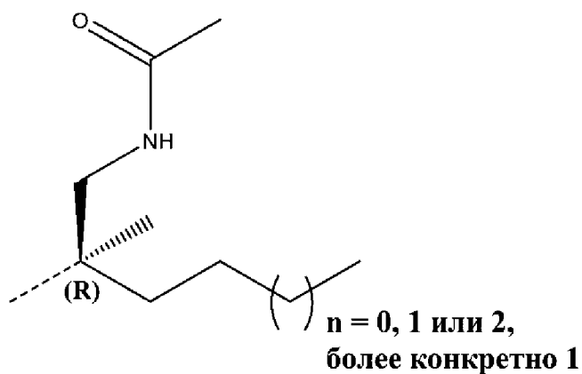
формула (V)
