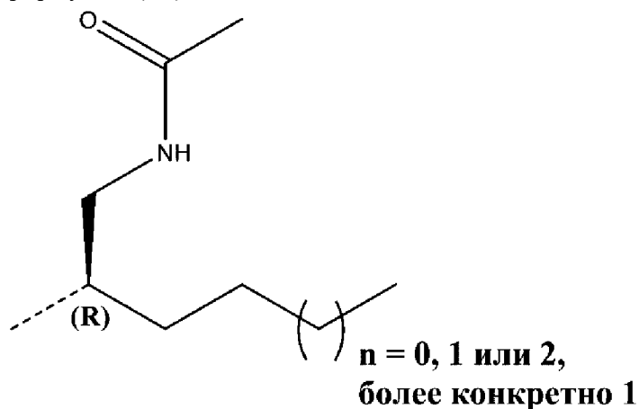
формула (IV)
