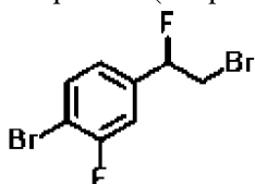
1-Бром-4-(2-бром-1-фторэтил)-2-фторбензол
