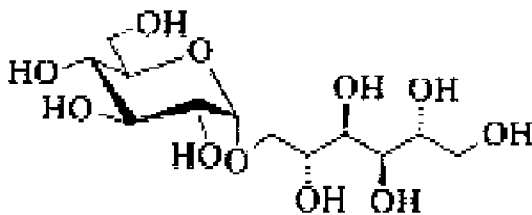
1- O - \alpha -D-Глюкопиранозил-D-маннит (1,1-GPM)
