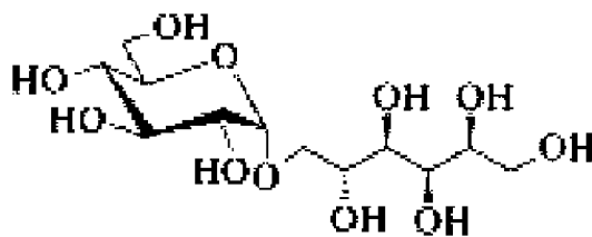
6- O - \alpha -D-Глюкопиранозил-D-сорбит (1,6-GPS)
